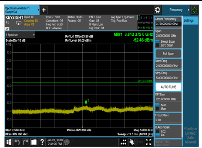
2480MHz,Plot 4,2500MHz~5000MHz
