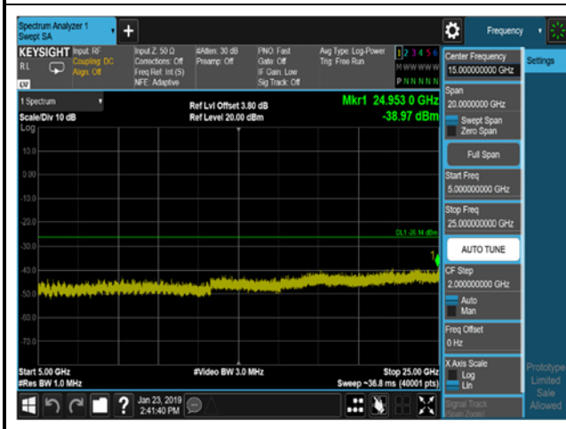
2480MHz,Plot 5,5000MHz~25000MHz
