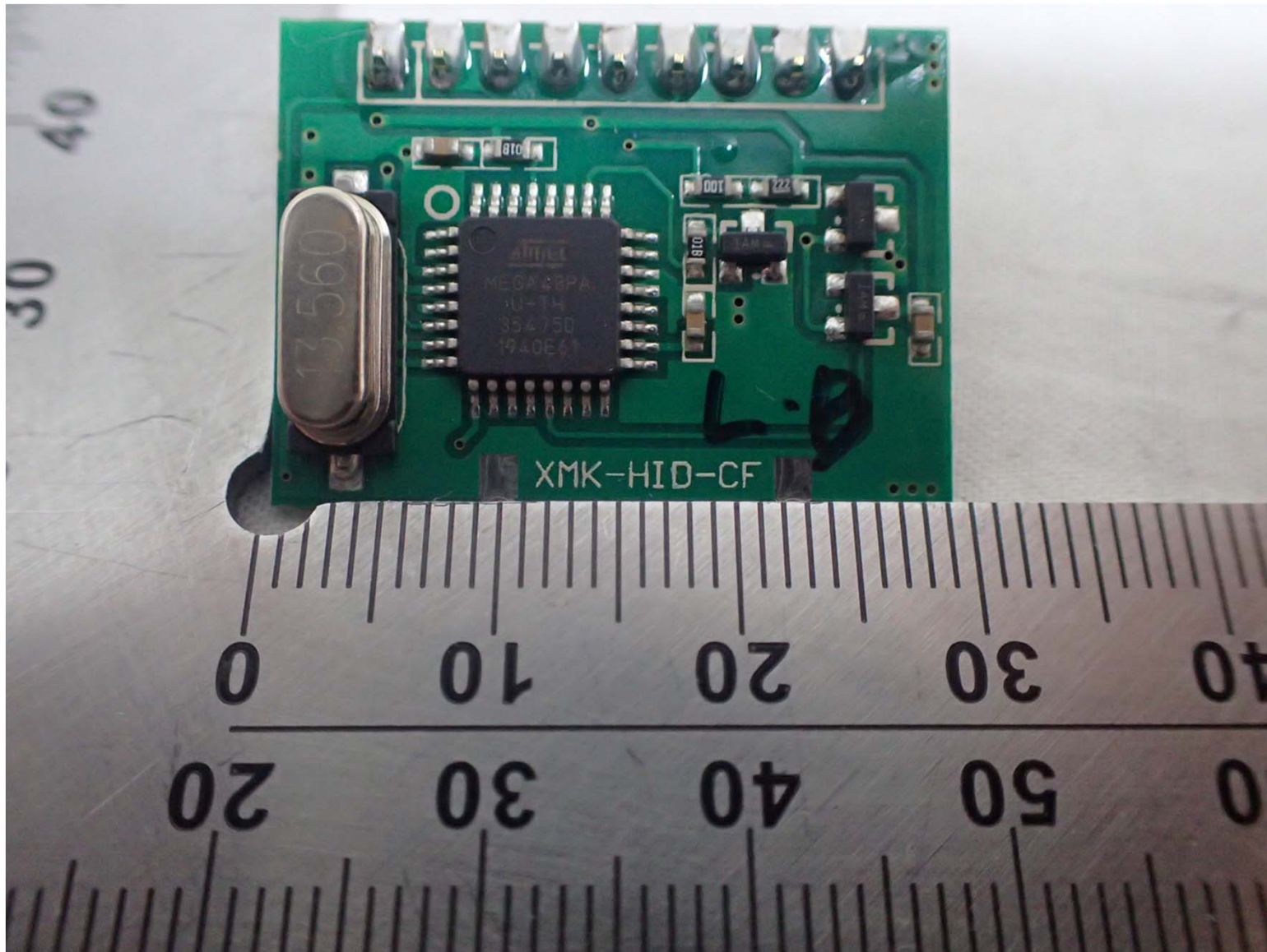
RF Module(RFID 125 kHz) Label
