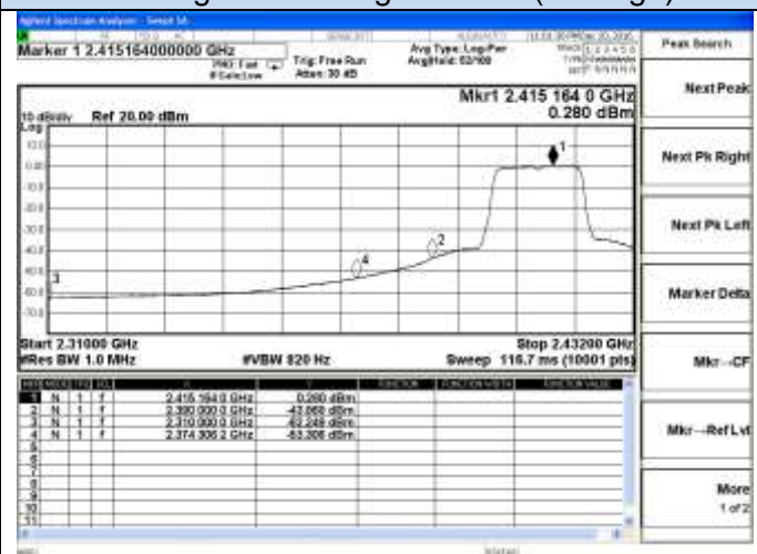
802.11n-HT20 Chain 0-Low channel(Average)
