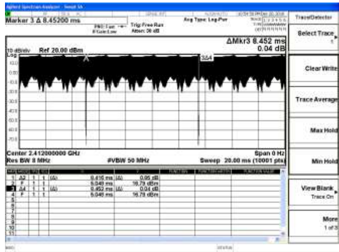
802.11b
