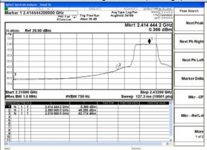
802.11g Chain 0-Low channel(Average)
