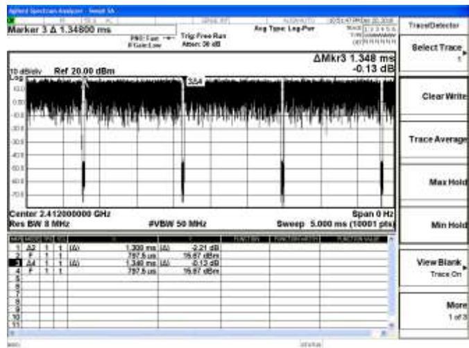
802.11n-HT20
