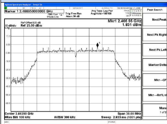
2447 – 2477 MHz
