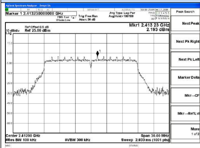
2397 – 2427 MHz
