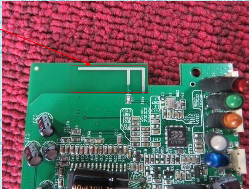
BT ANT
