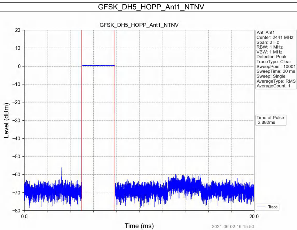
GFSK_DH5_HOPP_Ant1_NTNV
