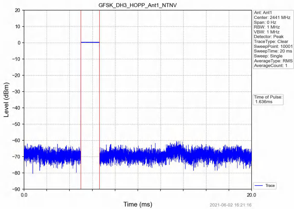
GFSK_DH3_HOPP_Ant1_NTNV
