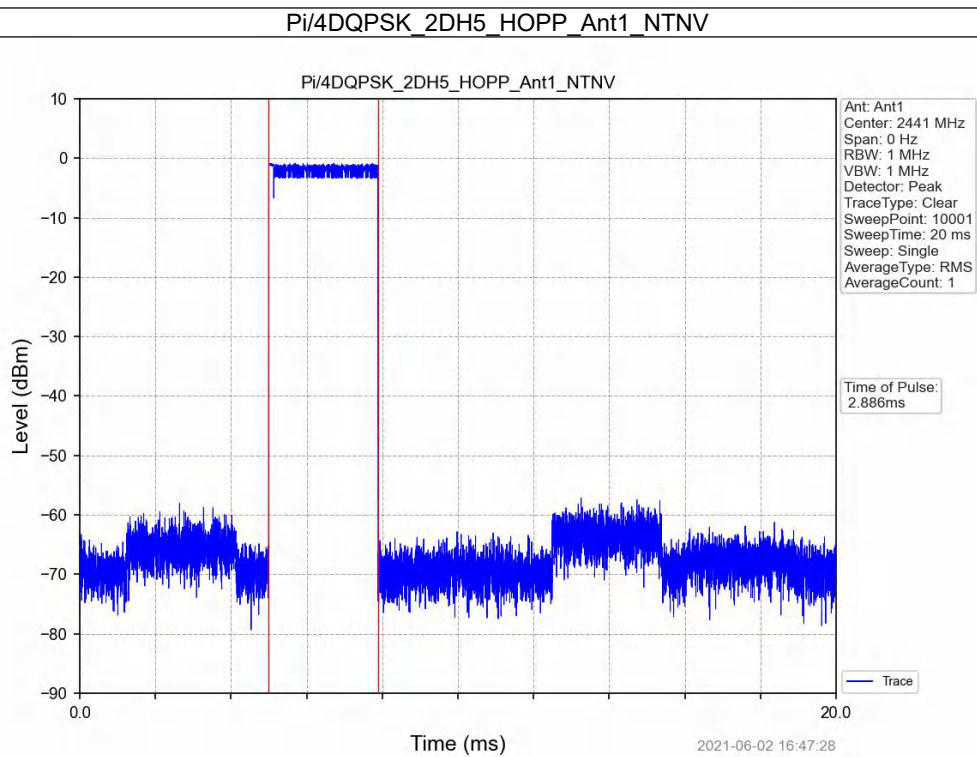
Pi/4DQPSK_2DH5_HOPP_Ant1_NTNV
