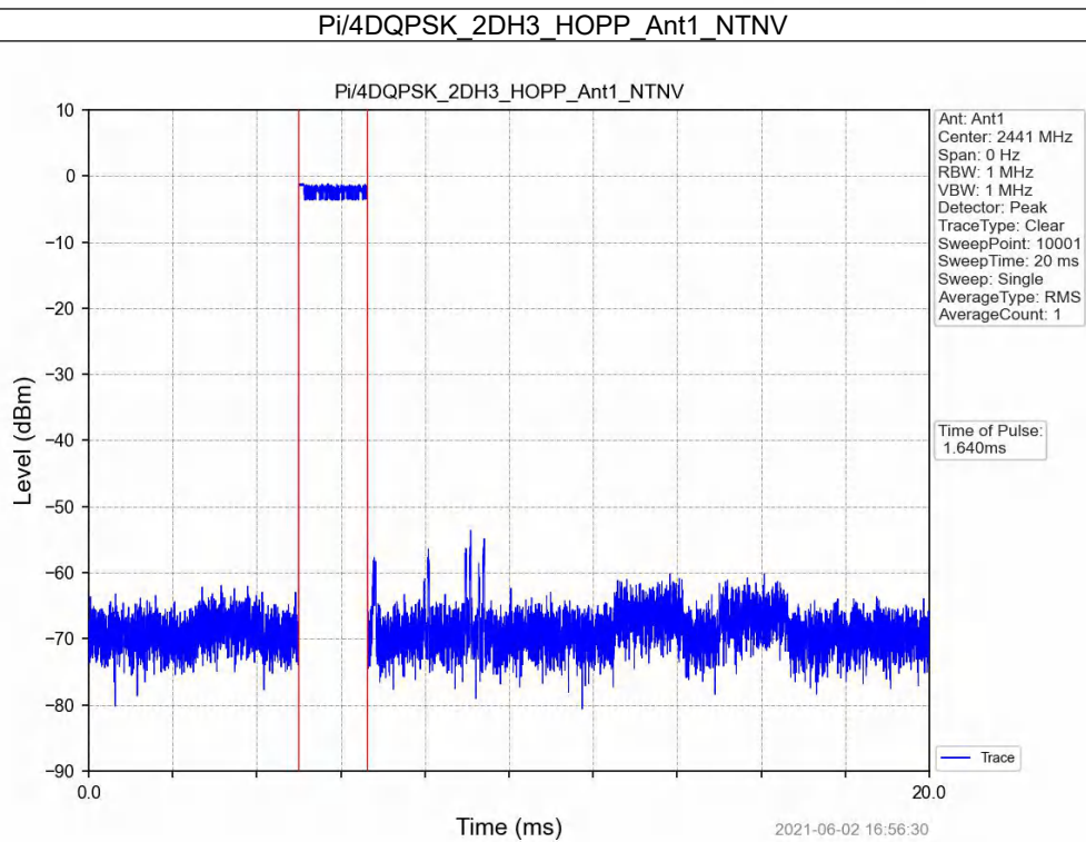
Pi/4DQPSK_2DH3_HOPP_Ant1_NTNV
