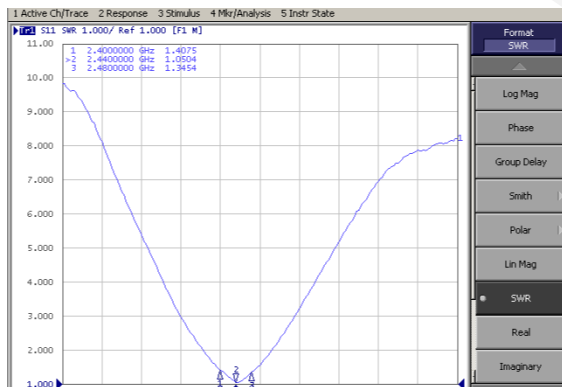
VSWR
