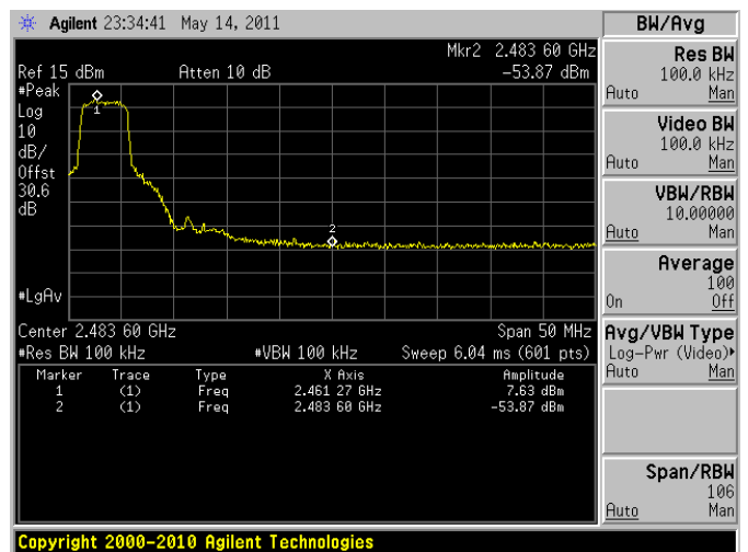
EIRP MIMO +36 dBm ~ High Band Edge
