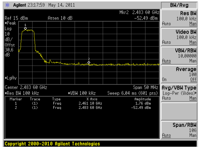
EIRP +30 dBm ~ High Band Edge
