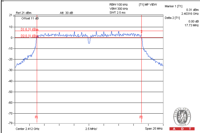
802.11n (20MHz)
