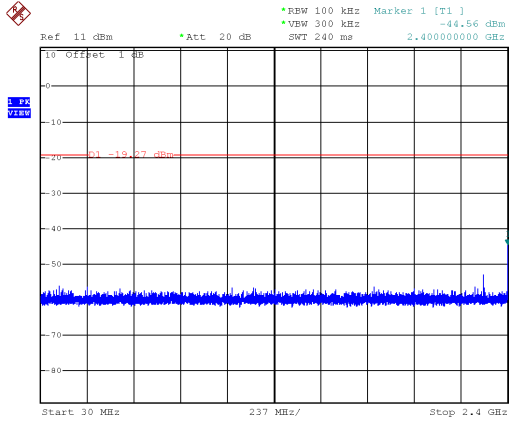
Modulation Type: \pi/4 DQPSK (2Mbps) CH00
