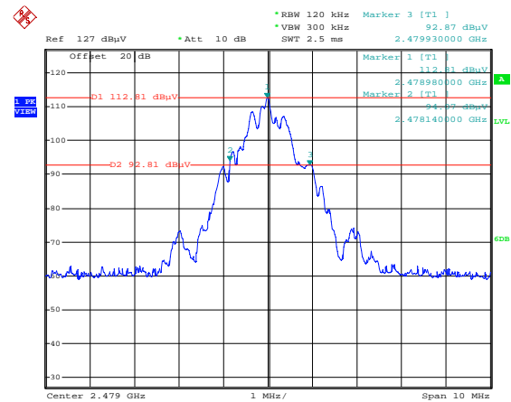
CH05, 2479MHz
