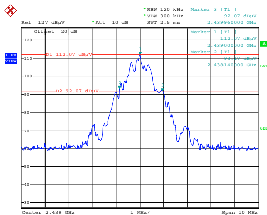
CH03, 2439MHz
