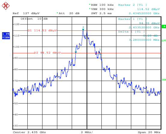
CH08, 2435MHz
