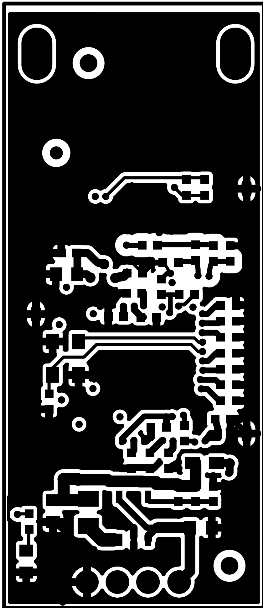
Bottom Layer
