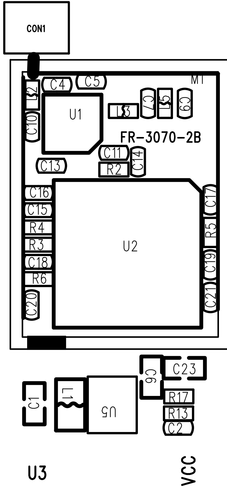
TopOverlay
