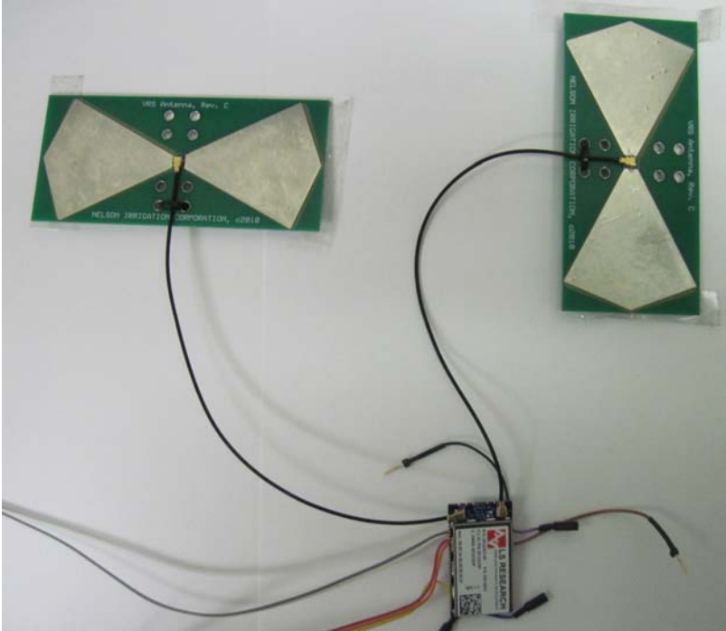
Nelson Bowtie Antenna
