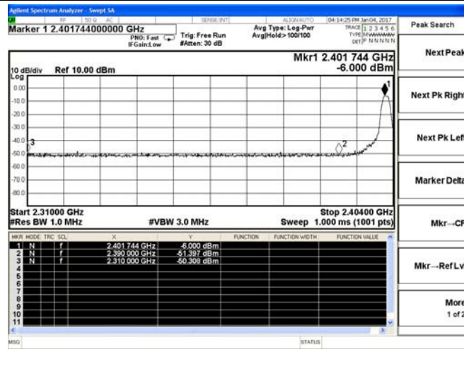
BLE 4.0-Low channel(Peak)
