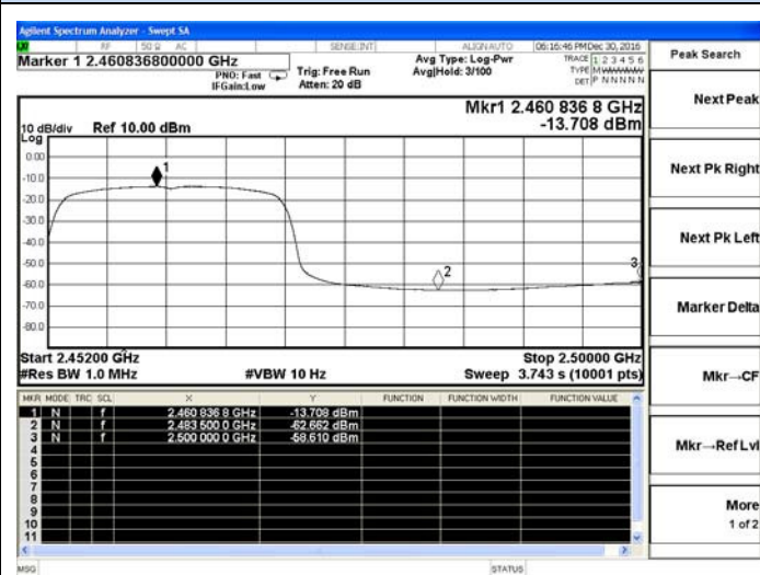
802.11n-HT20 High channel(Average)
