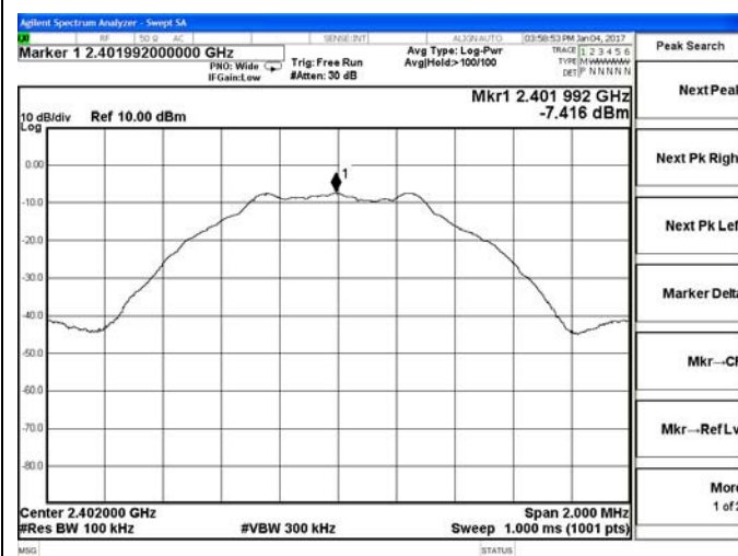
BLE 4.0_Low Channel
