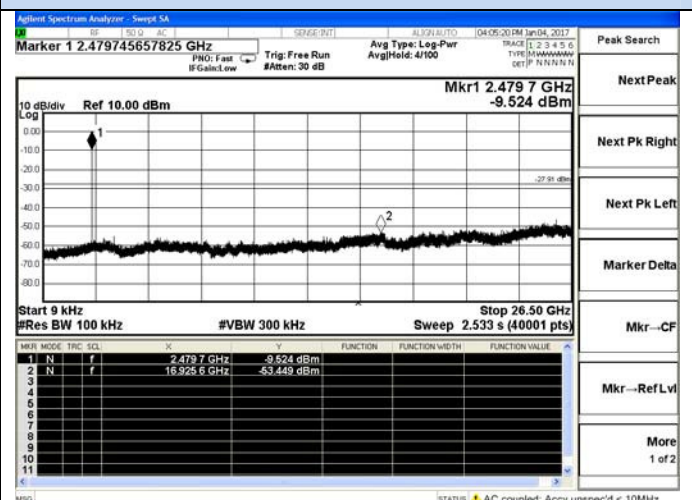
BLE 4.0-High channel
