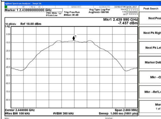
BLE 4.0-Middle channel Reference
