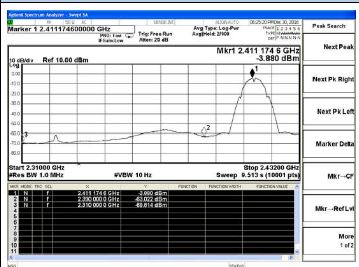
802.11b Low channel(Average)
