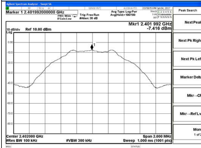
BLE 4.0-Low channel Reference
