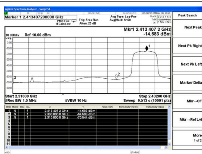
802.11n-HT20 Low channel(Average)
