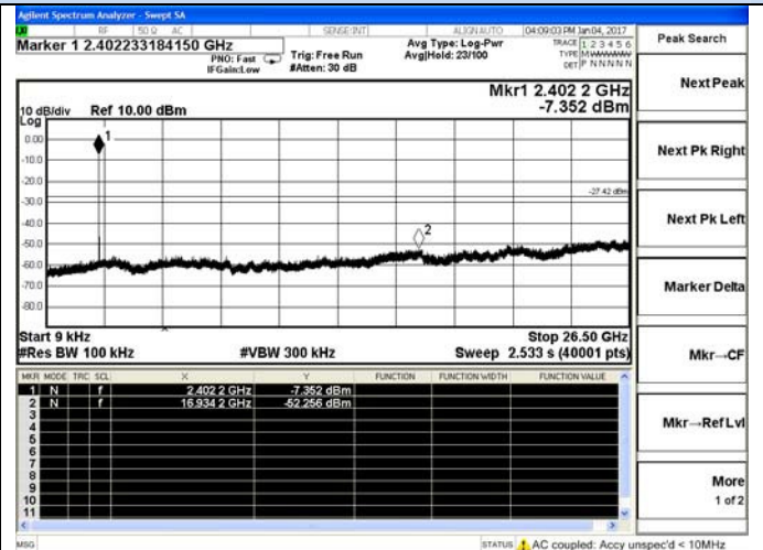
BLE 4.0-Low channel
