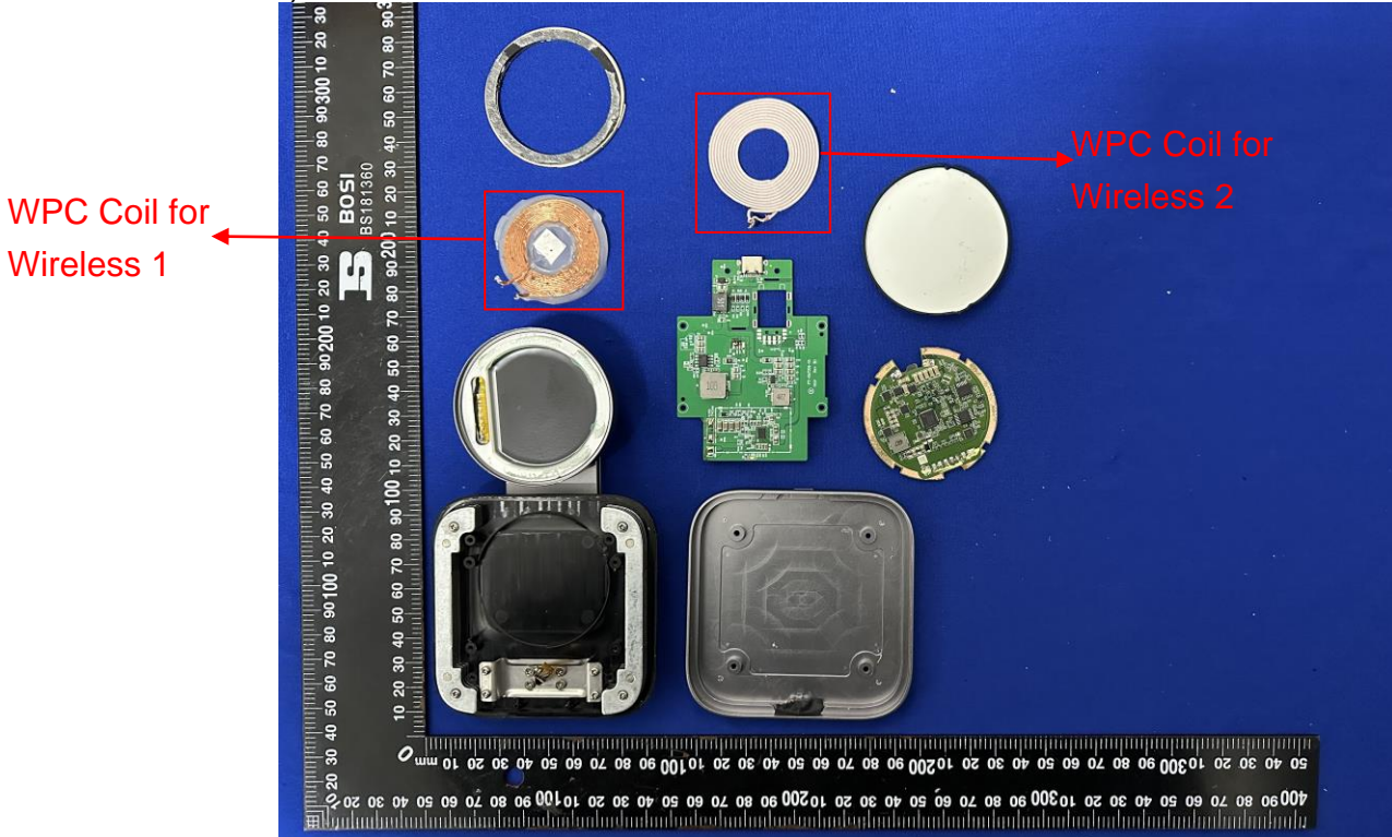
4) EUT Photo
