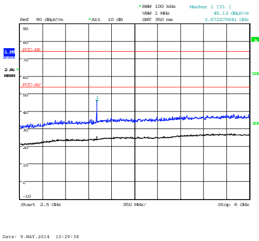
2.5GHz – 6GHz
