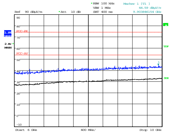
6GHz – 10GHz
