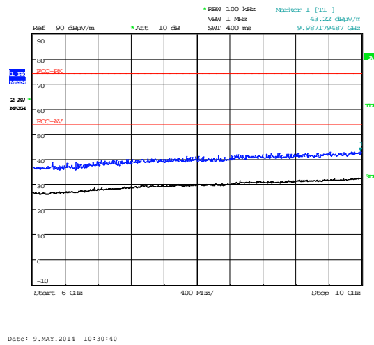
6GHz – 10GHz
