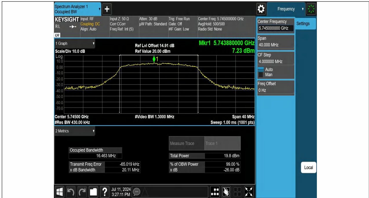
11A-Ant1-5745
