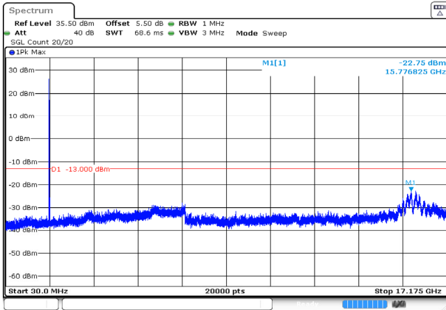
15MHz_Low_QPSK_1@0 -22.75dBm
