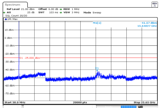
10MHz_High_QPSK_50@0 -41.57dBm
