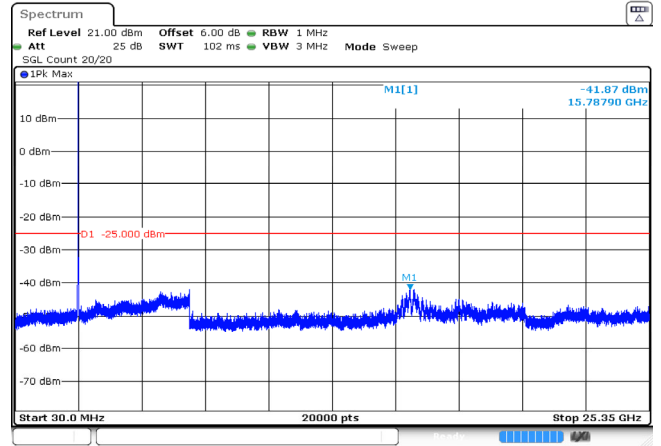
5MHz_Middle_QPSK_25@0 -41.87dBm
