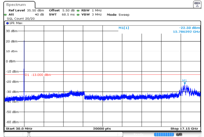
10MHz_Low_QPSK_50@0 -22.50dBm
