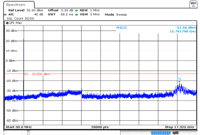
5MHz_Middle_QPSK_25@0 -21.66dBm
