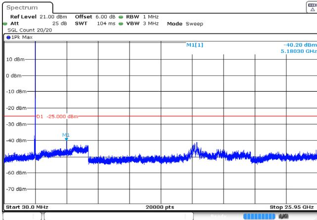
10MHz_Middle_QPSK_1@0 -40.20dBm
