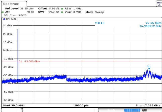
20MHz_Middle_QPSK_1@0 -22.96dBm
