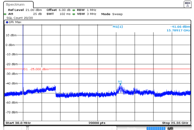
15MHz_Middle_QPSK_75@0 -41.66dBm
