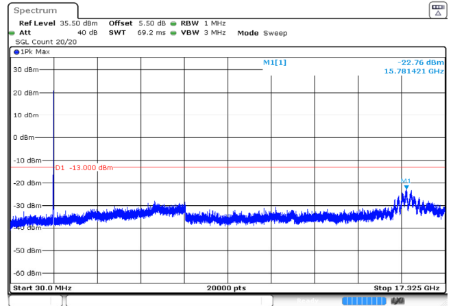
10MHz_Middle_QPSK_50@0 -22.76dBm
