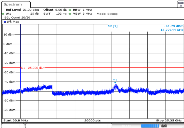
20MHz_Middle_QPSK_1@0 -41.79dBm
