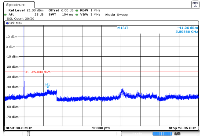
10MHz_Middle_QPSK_50@0 -41.36dBm
