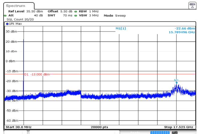
5MHz_High_QPSK_25@0 -22.66dBm
