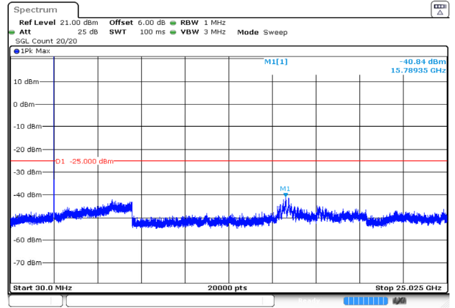
5MHz_Low_QPSK_25@0 -40.84dBm
