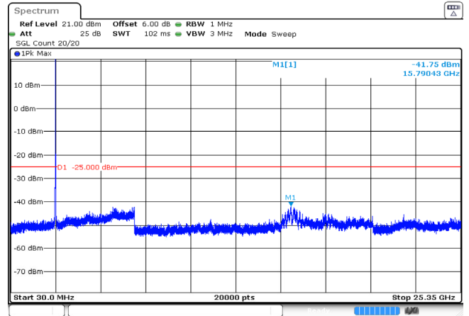
10MHz_Middle_QPSK_50@0 -41.75dBm
