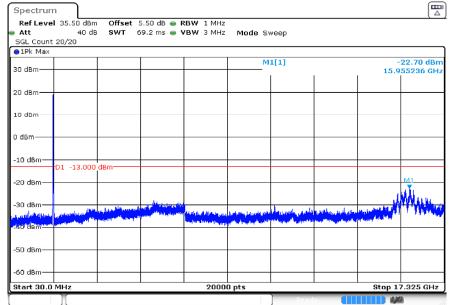
20MHz_Middle_QPSK_100@0 -22.70dBm
