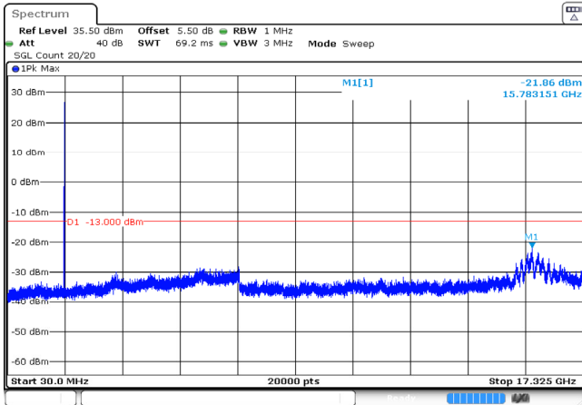
10MHz_Middle_QPSK_1@0 -21.86dBm
