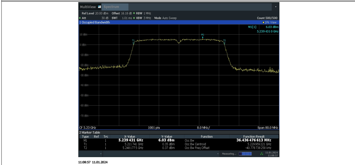
11N40MIMO_Ant10_5230
