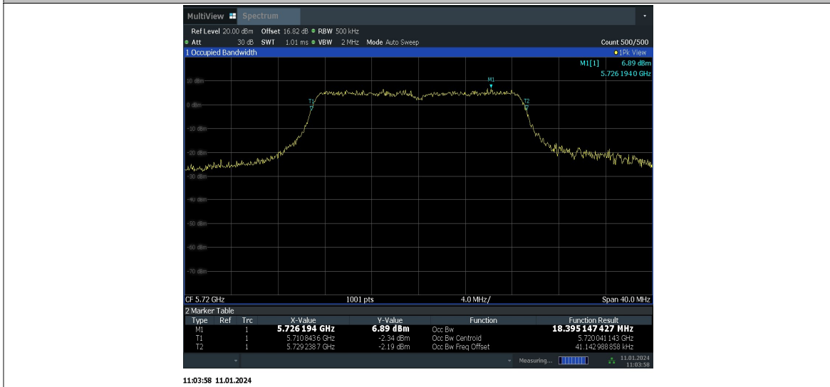
11N20MIMO_Ant10_5720
