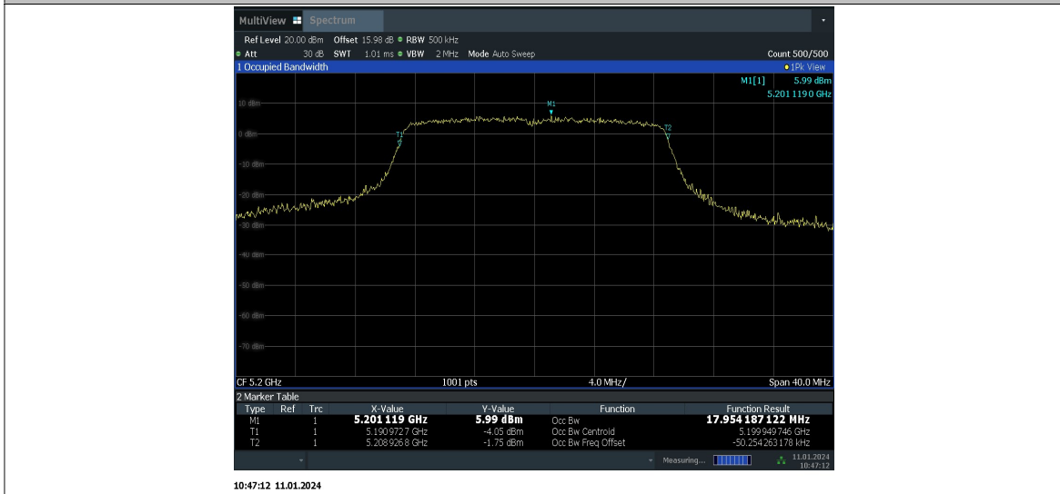
11N20MIMO_Ant10_5200
