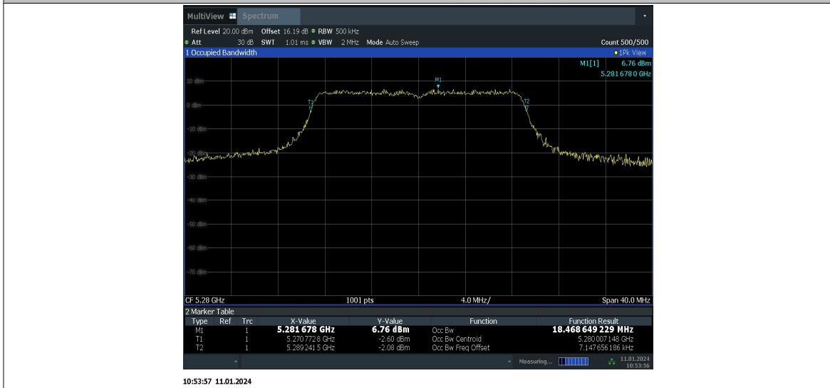
11N20MIMO_Ant10_5280
