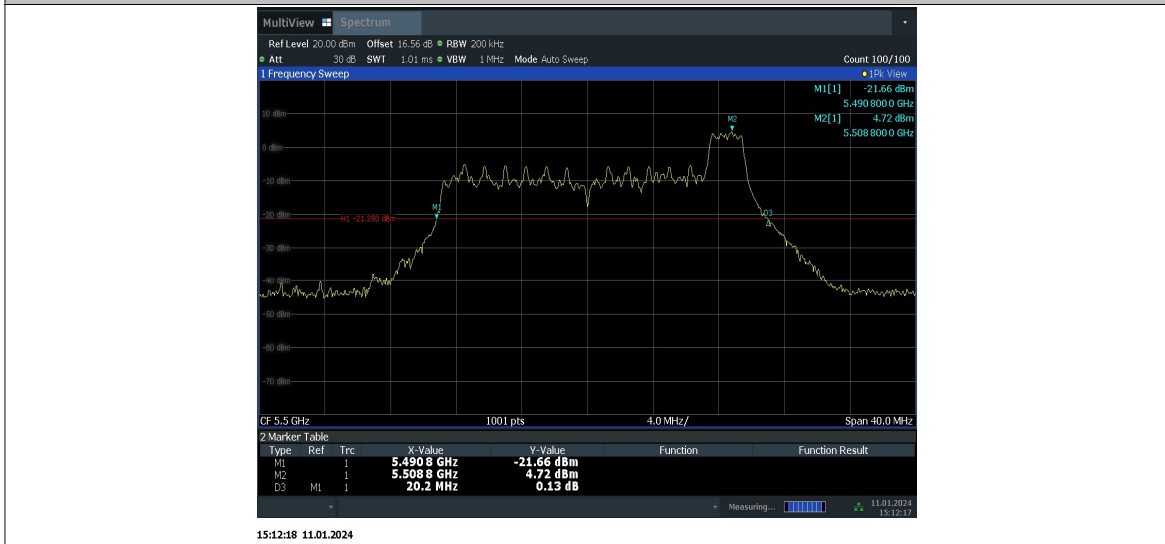
11AX20MIMO_Ant6_5500_52Tone_RU40
