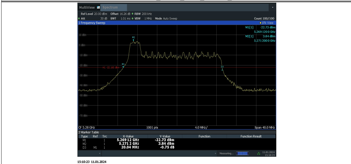
11AX20MIMO_Ant10_5280_26Tone_RU0
