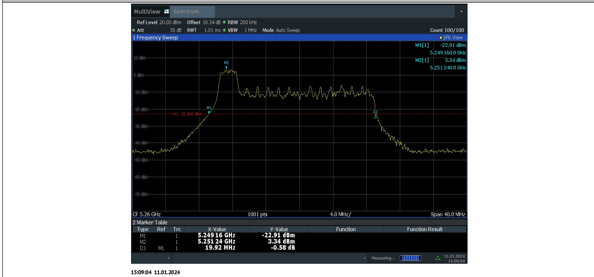
11AX20MIMO_Ant10_5260_52Tone_RU37
