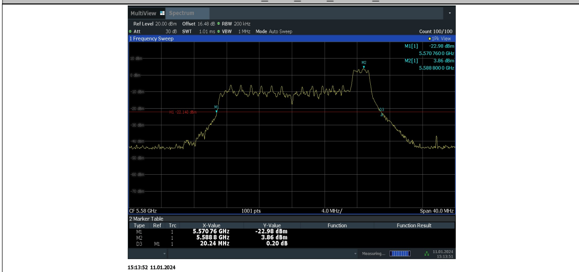
11AX20MIMO_Ant6_5580_26Tone_RU8
