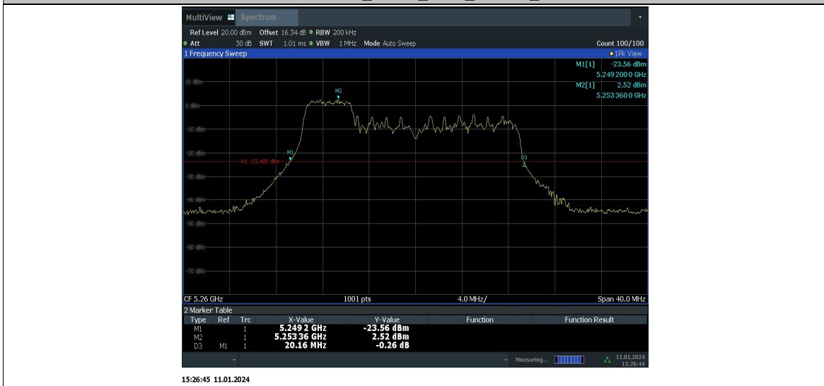
11AX20MIMO_Ant10_5260_52Tone_RU37
