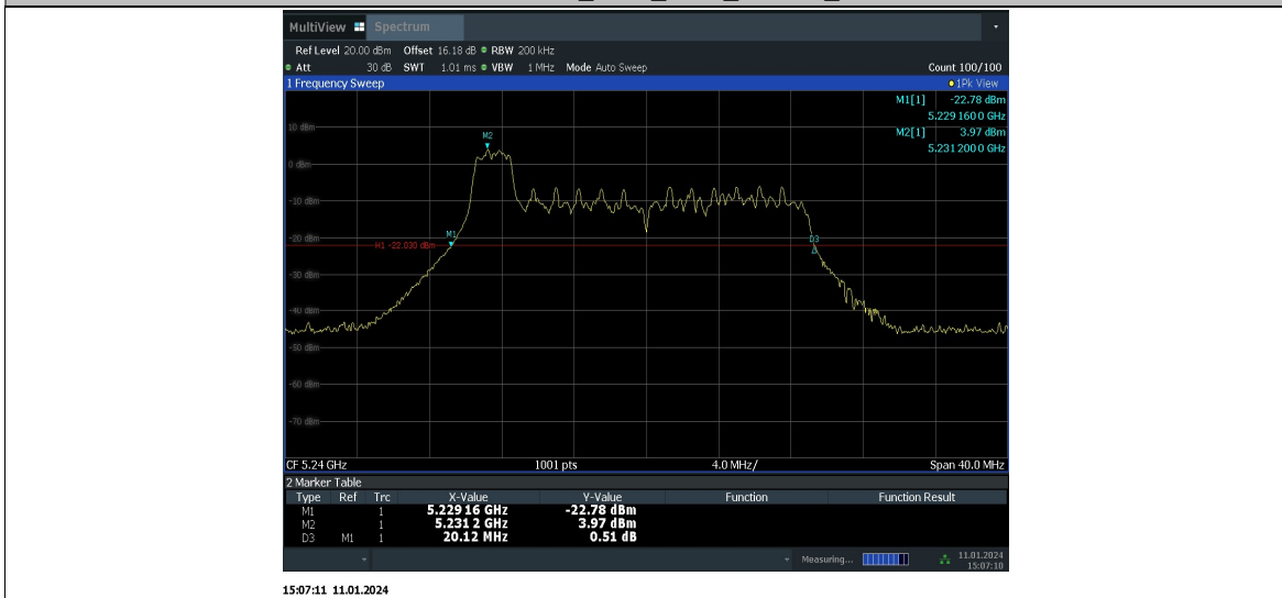
11AX20MIMO_Ant6_5240_26Tone_RU0
