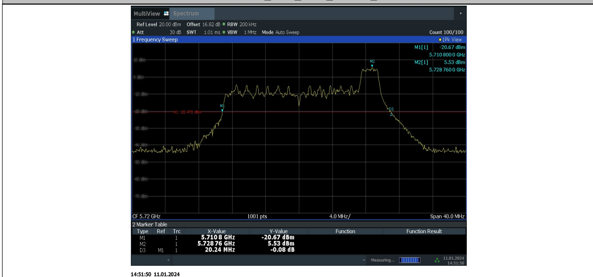
11AX20SISO_Ant6_5720_26Tone_RU8
