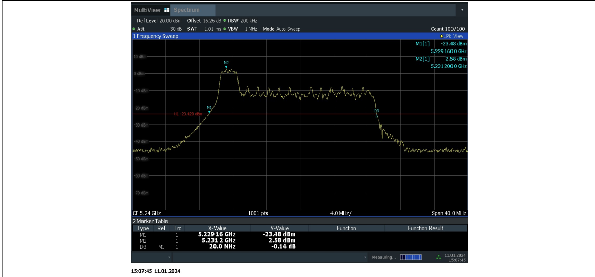
11AX20MIMO_Ant10_5240_52Tone_RU37
