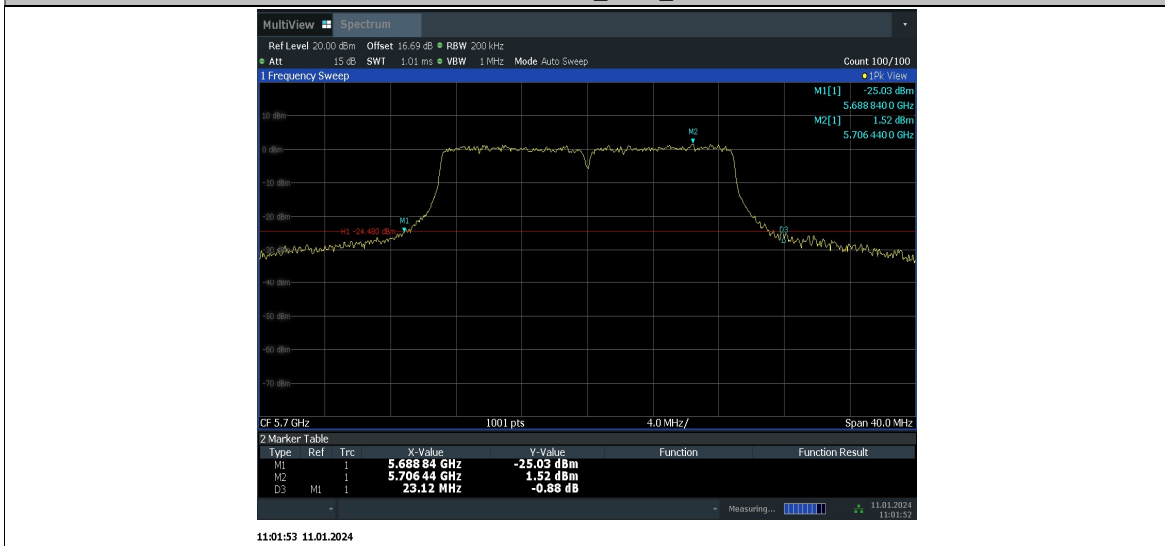
11N20MIMO_Ant6_5700
