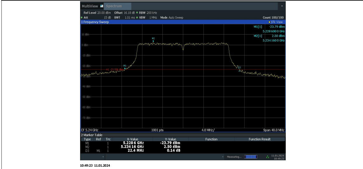
11N20MIMO_Ant10_5240
