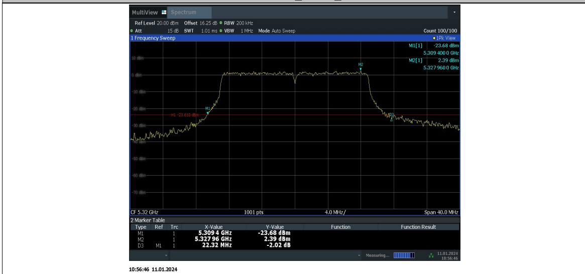
11N20MIMO_Ant10_5320
