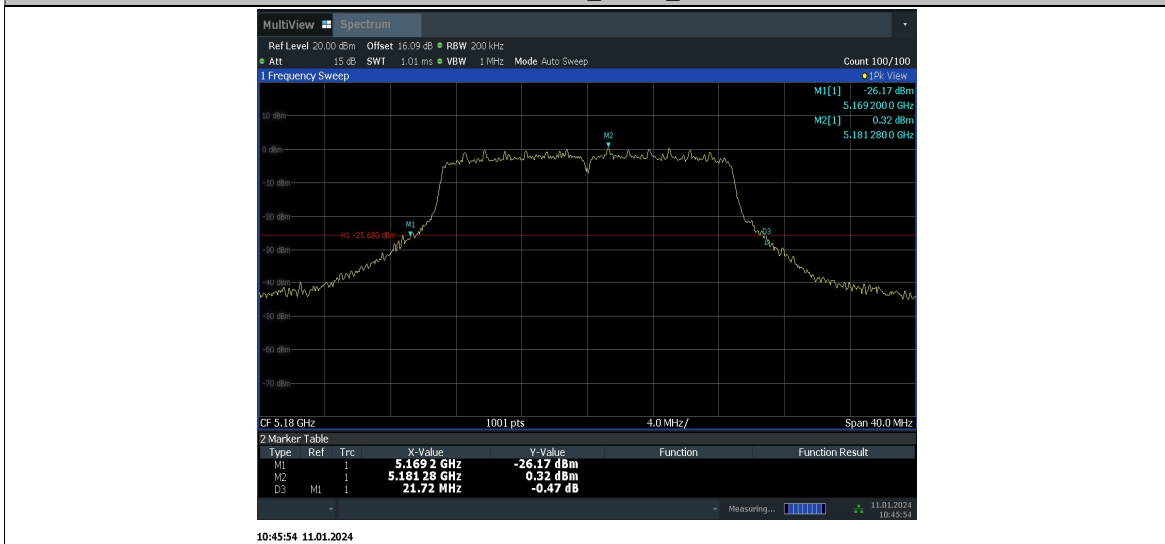
11N20MIMO_Ant10_5180
