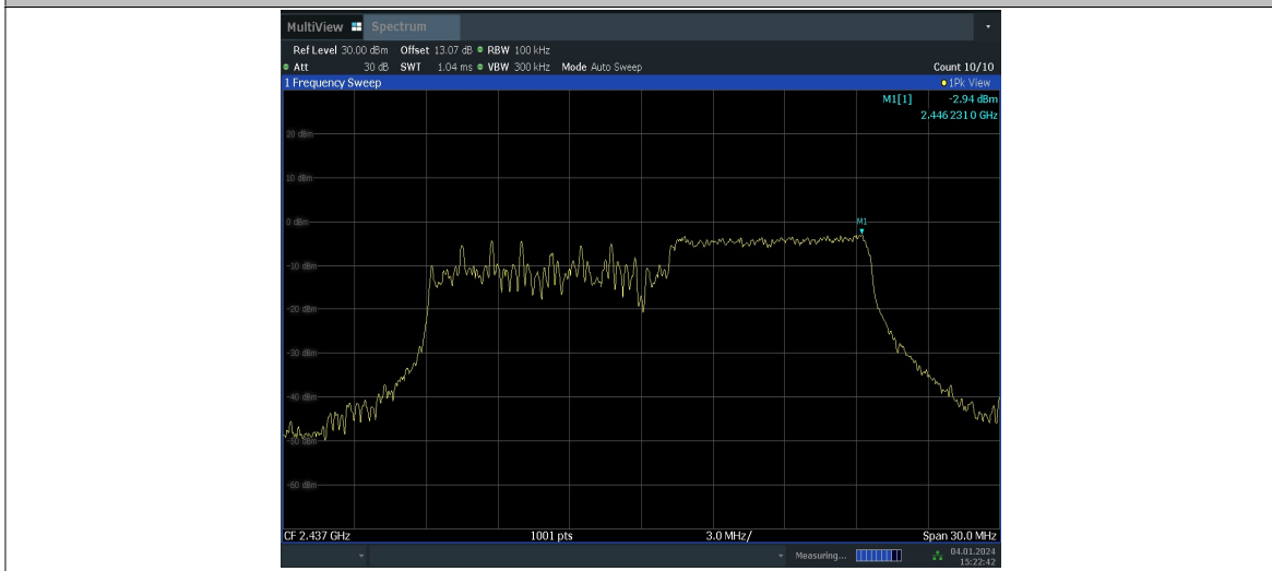
11AX20MIMO_Ant10_2437_106Tone_RU54_0~Reference
