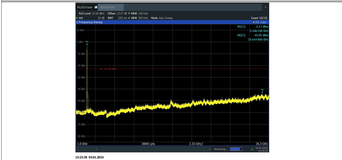
11AX20MIMO_Ant6_2462_26Tone_RU0_0~Reference
