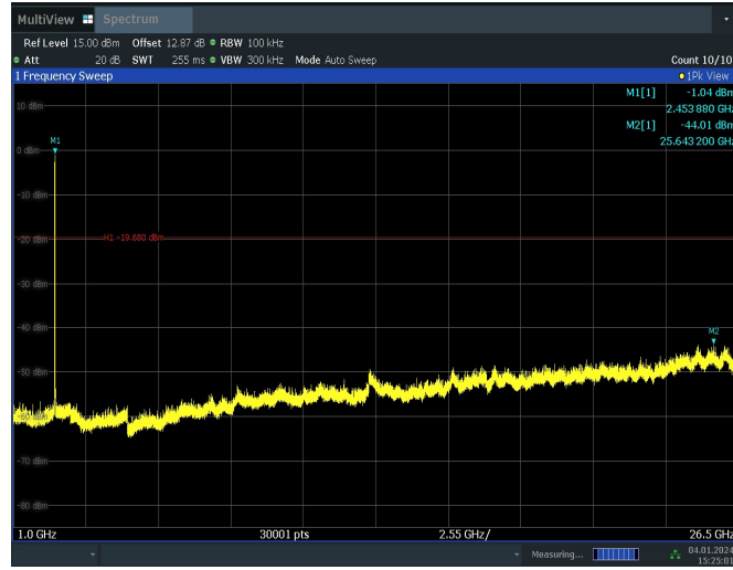
11AX20MIMO_Ant6_2462_26Tone_RU8_0~Reference
