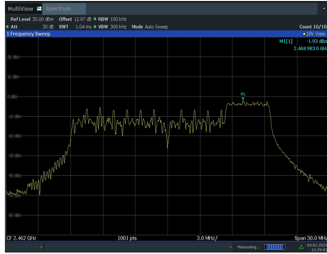
11AX20MIMO_Ant6_2462_52Tone_RU40_0-Reference
