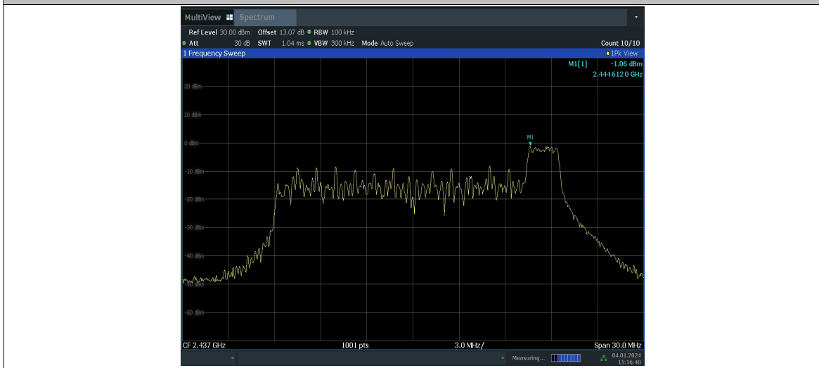
11AX20MIMO_Ant10_2437_26Tone_RU8_0-Reference
