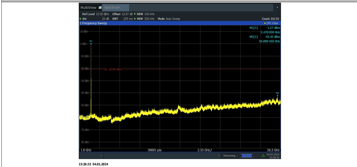
11AX20MIMO_Ant6_2462_52Tone_RU37_0~Reference
