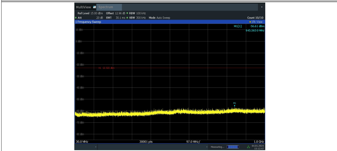
11AX20MIMO_Ant6_2437_106Tone_RU53_30~1000
