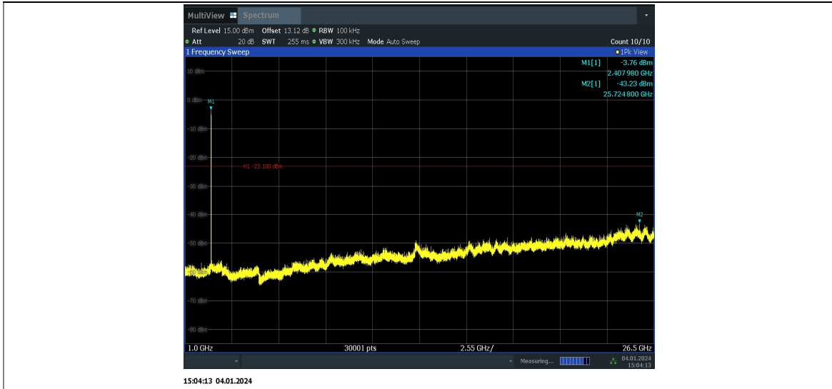
11AX20MIMO_Ant10_2412_106Tone_RU54_0~Reference
