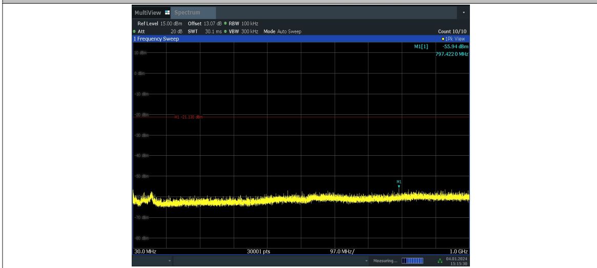
11AX20MIMO_Ant10_2437_26Tone_RU0_30~1000
