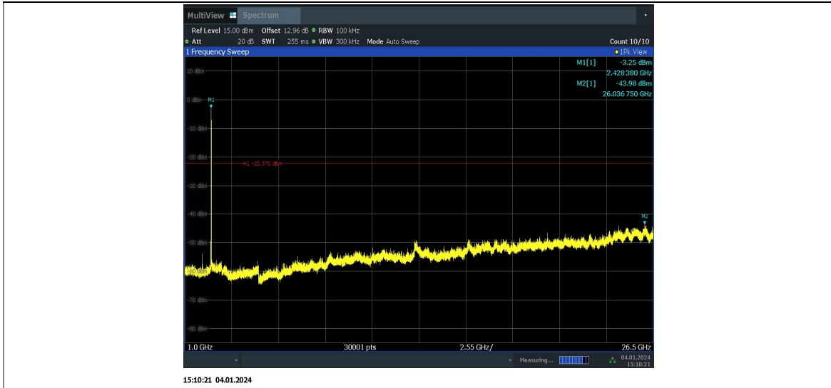
11AX20MIMO_Ant6_2437_52Tone_RU40_0-Reference
