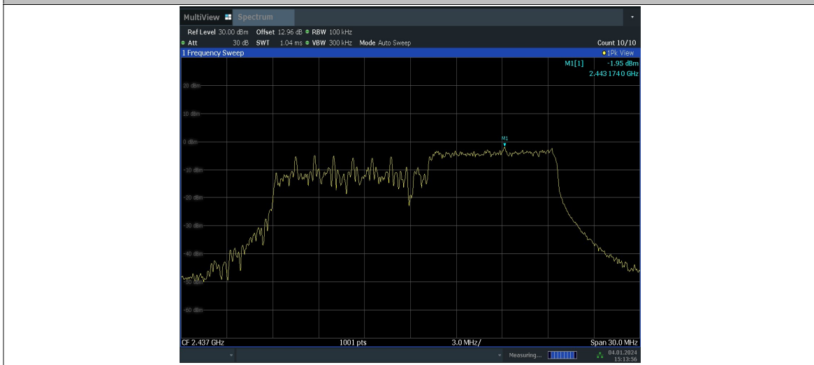
11AX20MIMO_Ant6_2437_106Tone_RU54_0~Reference
