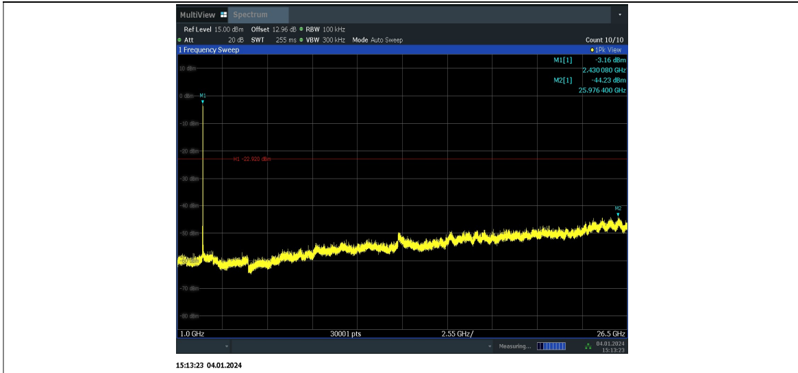
11AX20MIMO_Ant6_2437_106Tone_RU54_0~Reference
