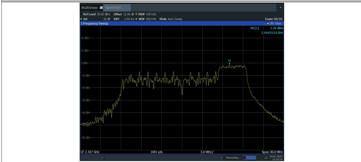
11AX20MIMO_Ant6_2437_52Tone_RU40_0-Reference
