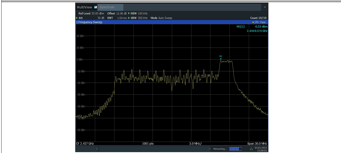
11AX20MIMO_Ant6_2437_26Tone_RU8_0~Reference
