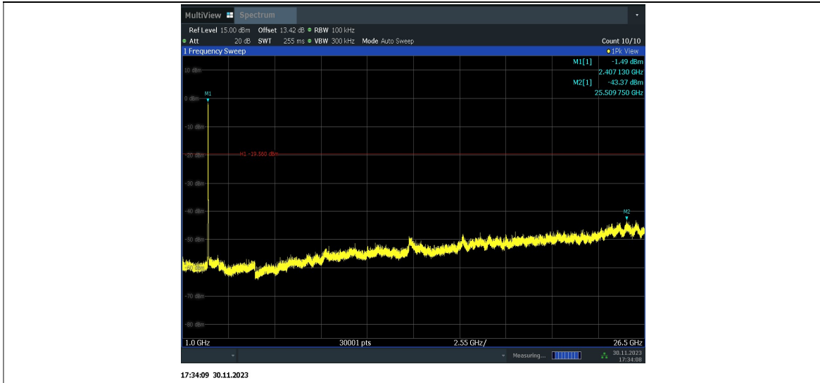
11N20MIMO_Ant10_2412_0-Reference
