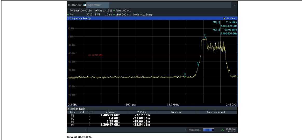
11AX20MIMO_Ant10_Low_2412_52Tone_RU40
