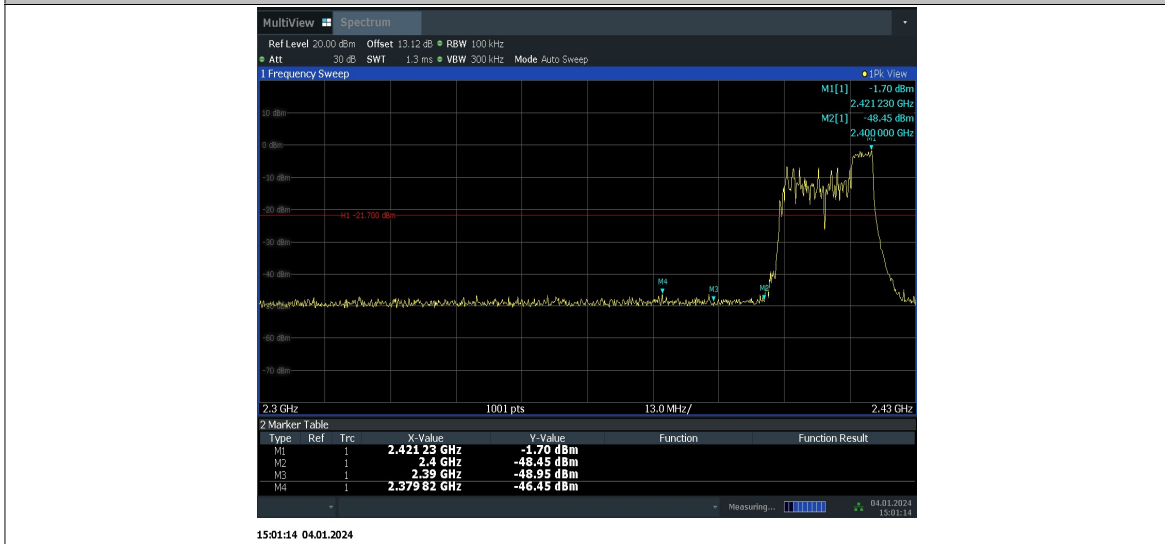
11AX20MIMO_Ant10_Low_2412_106Tone_RU53
