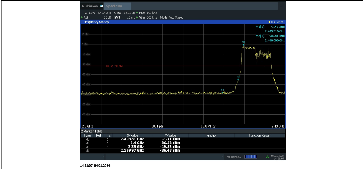
11AX20MIMO_Ant6_Low_2412_106Tone_RU54
