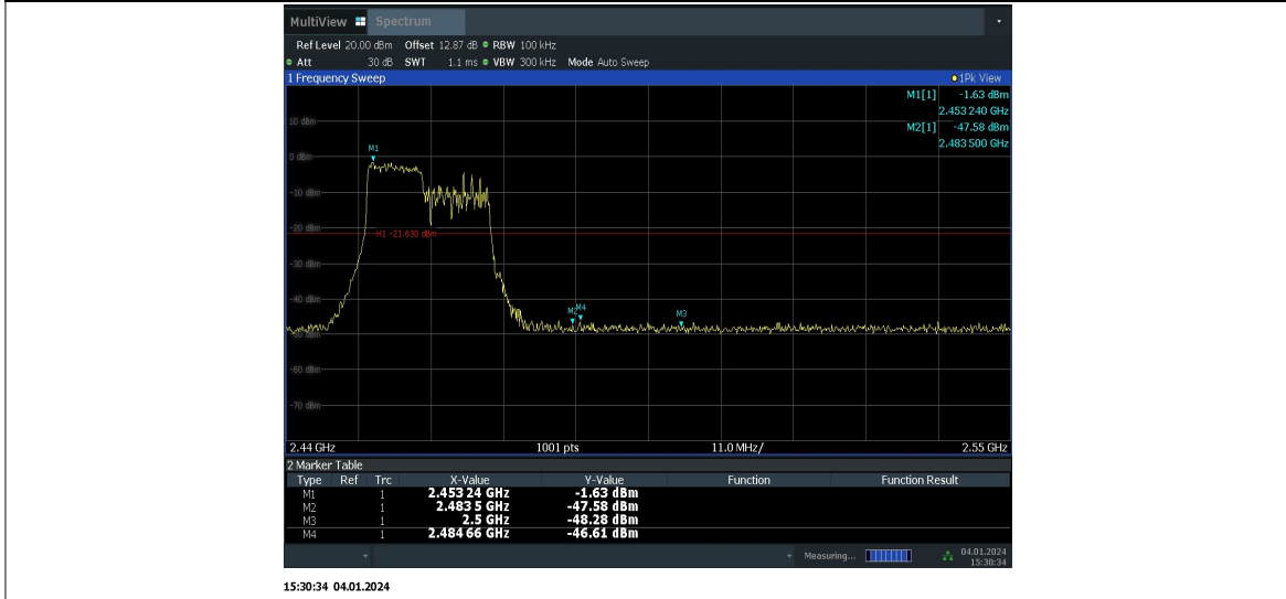
11AX20MIMO_Ant6_High_2462_106Tone_RU54
