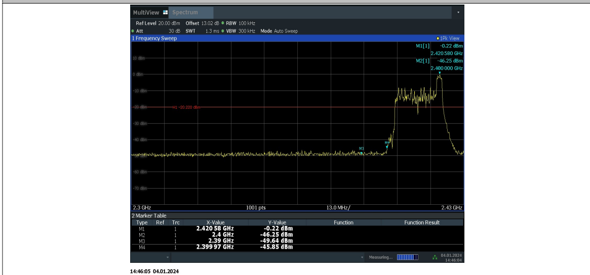
11AX20MIMO_Ant6_Low_2412_52Tone_RU37
