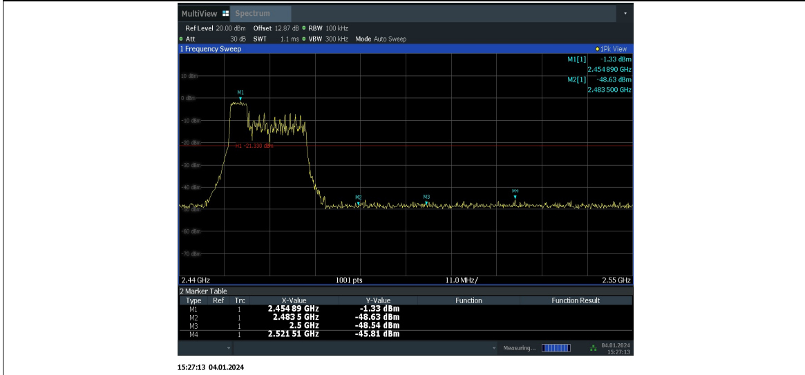
11AX20MIMO_Ant6_High_2462_52Tone_RU40
