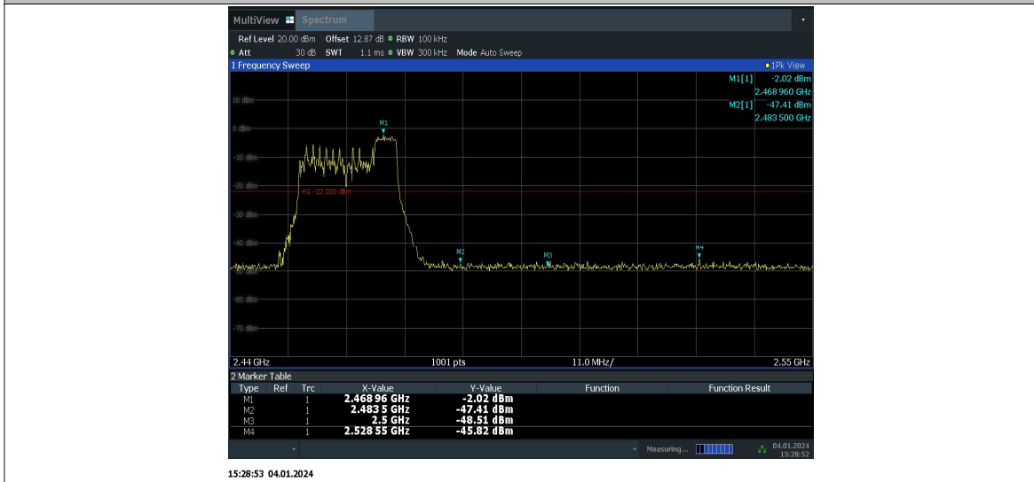
11AX20MIMO_Ant6_High_2462_106Tone_RU53
