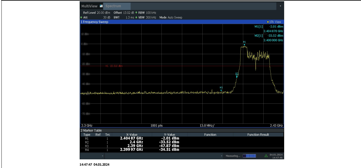
11AX20MIMO_Ant6_Low_2412_52Tone_RU40
