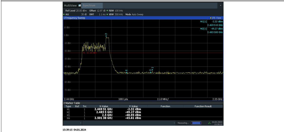
11AX20MIMO_Ant10_High_2462_52Tone_RU37
