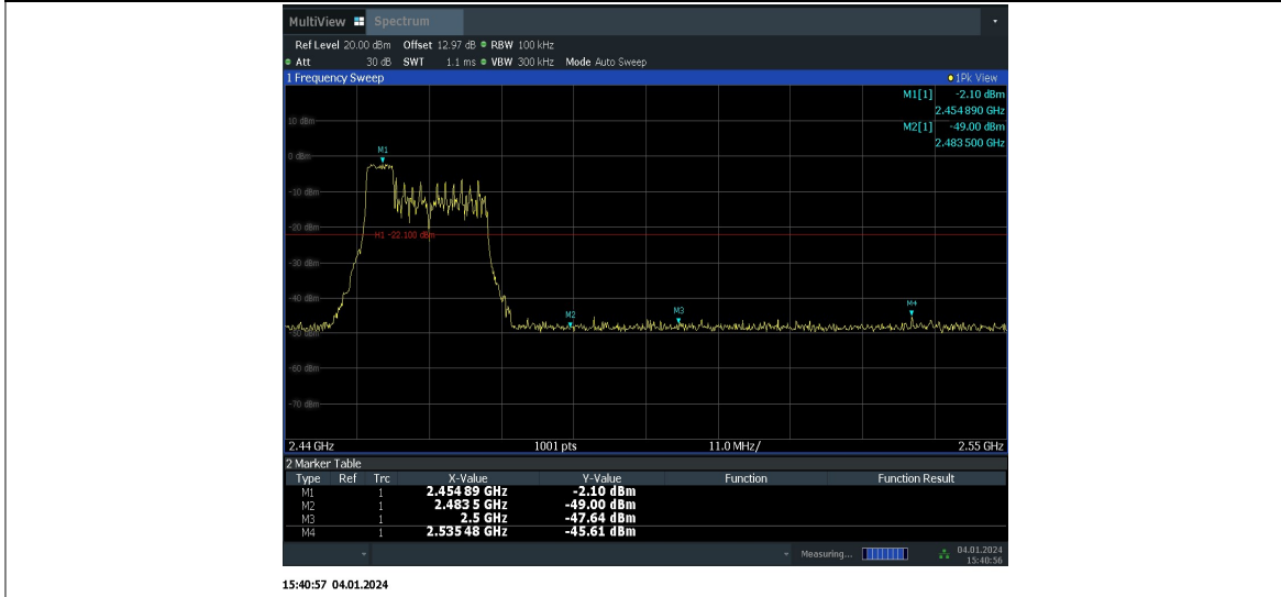
11AX20MIMO_Ant10_High_2462_52Tone_RU40
