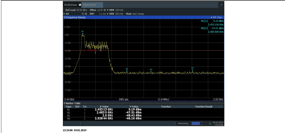
11AX20MIMO_Ant6_High_2462_26Tone_RU8
