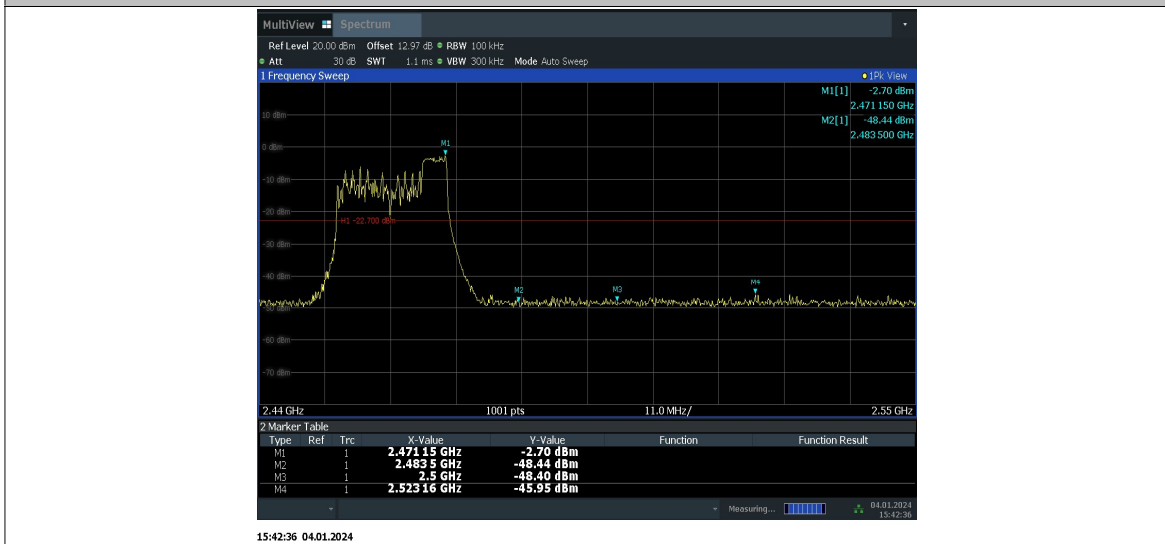
11AX20MIMO_Ant10_High_2462_106Tone_RU53
