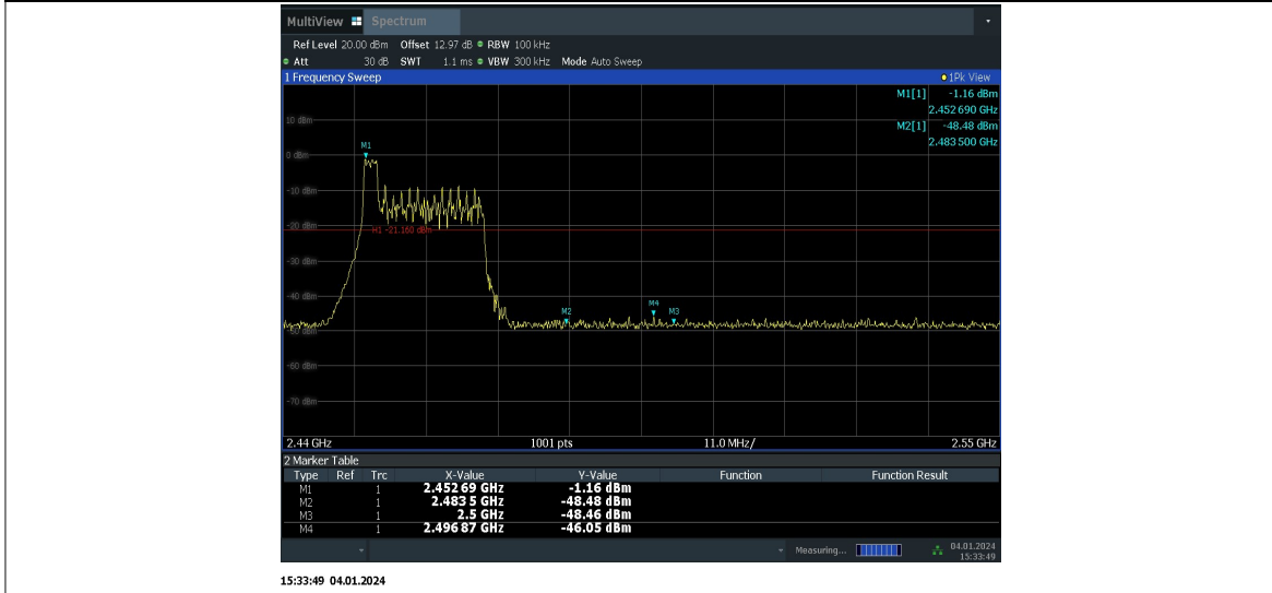
11AX20MIMO_Ant10_High_2462_26Tone_RU8
