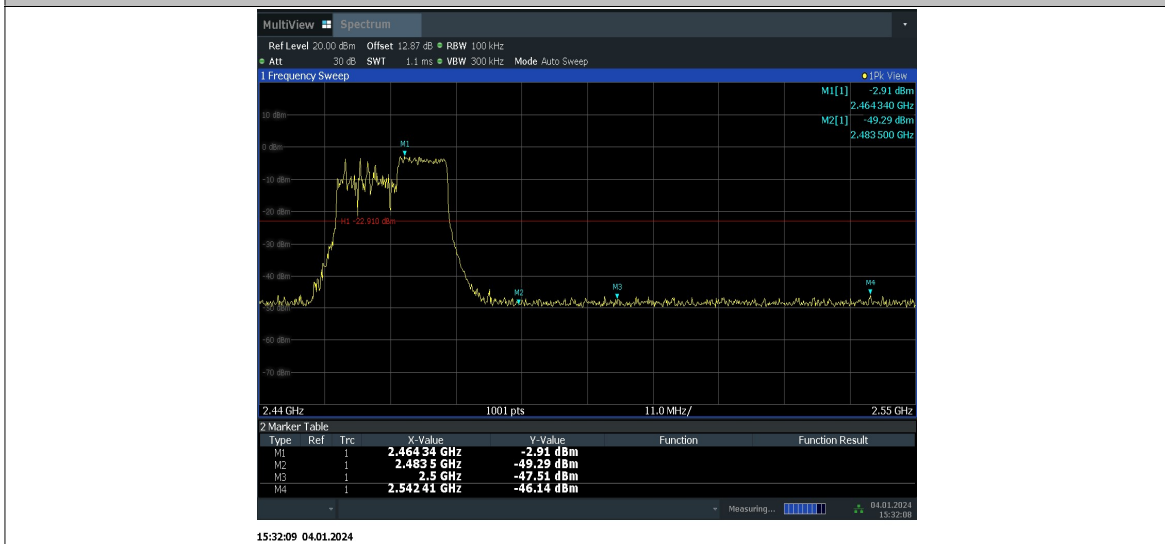
11AX20MIMO_Ant10_High_2462_26Tone_RU0
