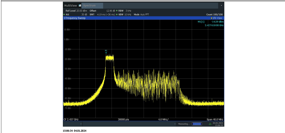
11AX20MIMO_Ant6_2437_26Tone_RU8
