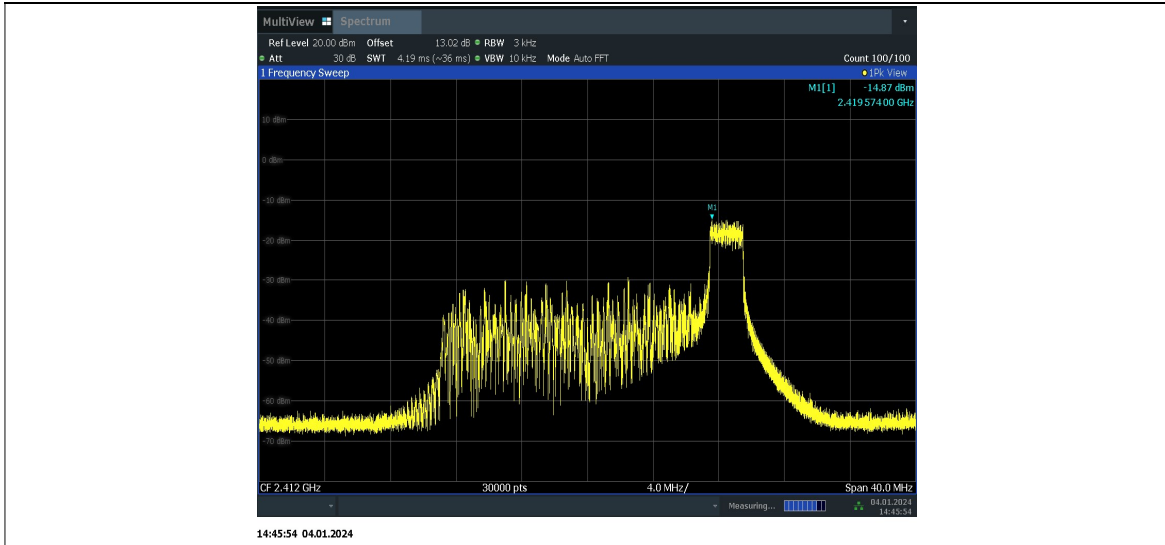
11AX20MIMO_Ant6_2412_52Tone_RU37
