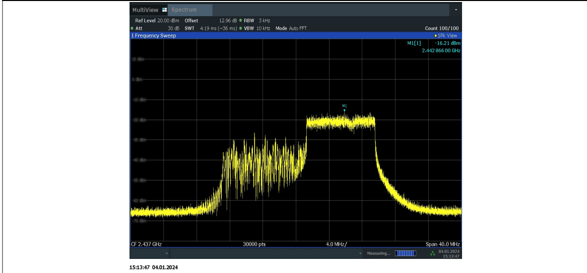
11AX20MIMO_Ant10_2437_26Tone_RU0
