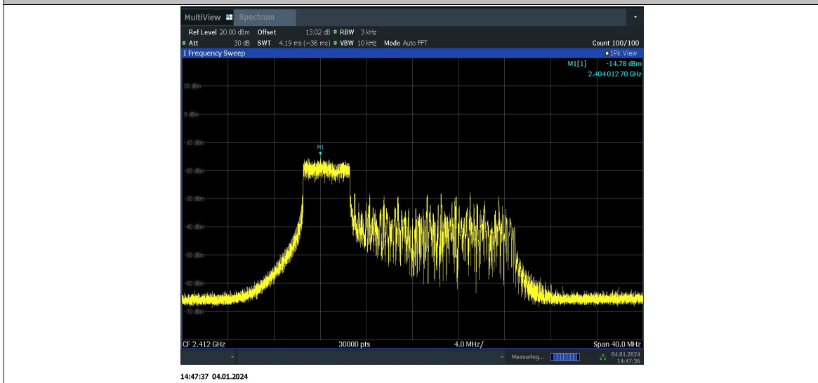
11AX20MIMO_Ant6_2412_52Tone_RU40
