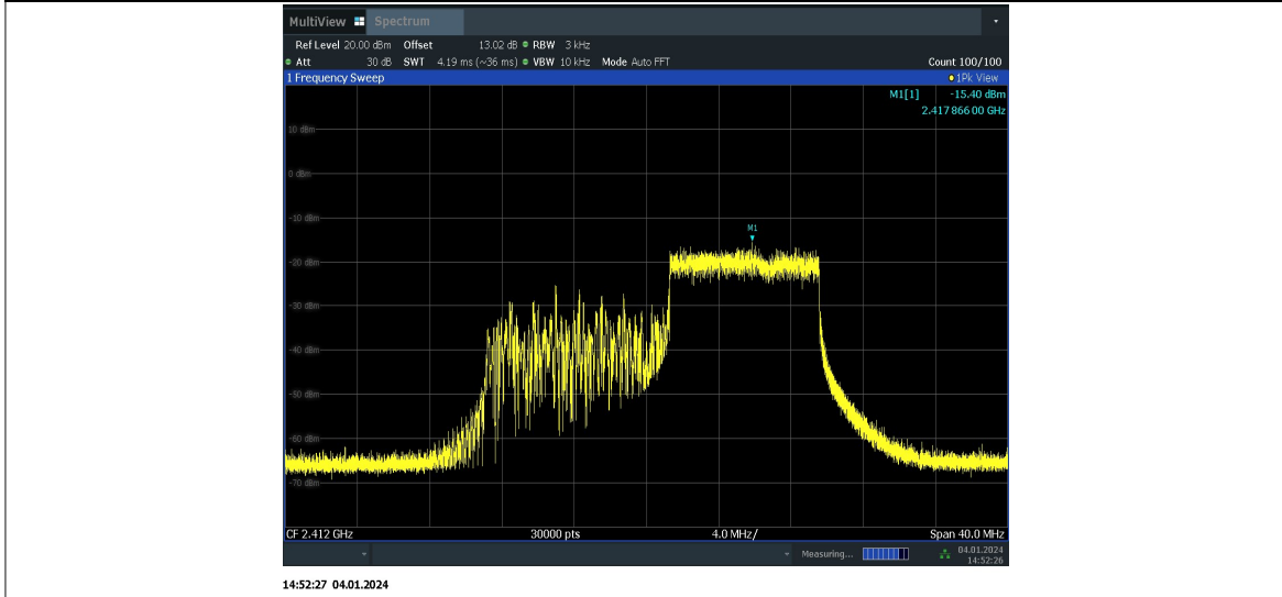
11AX20MIMO_Ant10_2412_26Tone_RU0
