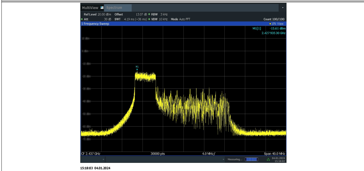
11AX20MIMO_Ant10_2437_52Tone_RU40
