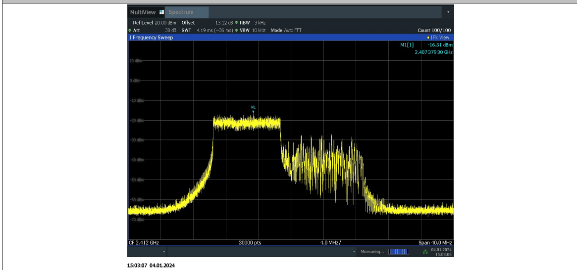
11AX20MIMO_Ant10_2412_106Tone_RU54
