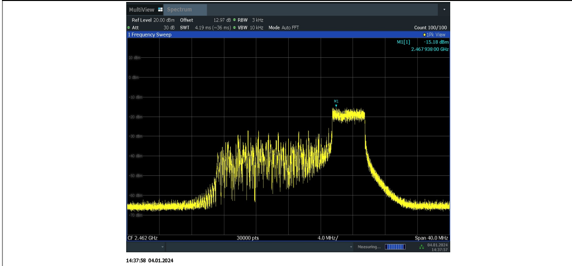
11AX20SISO_Ant10_2462_106Tone_RU53
