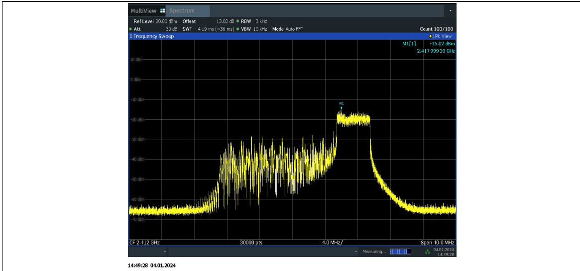
11AX20MIMO_Ant6_2412_106Tone_RU53
