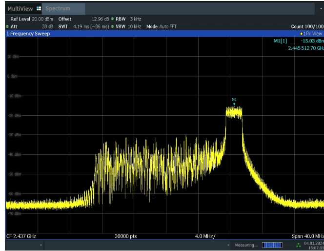
11AX20MIMO_Ant6_2437_52Tone_RU37
