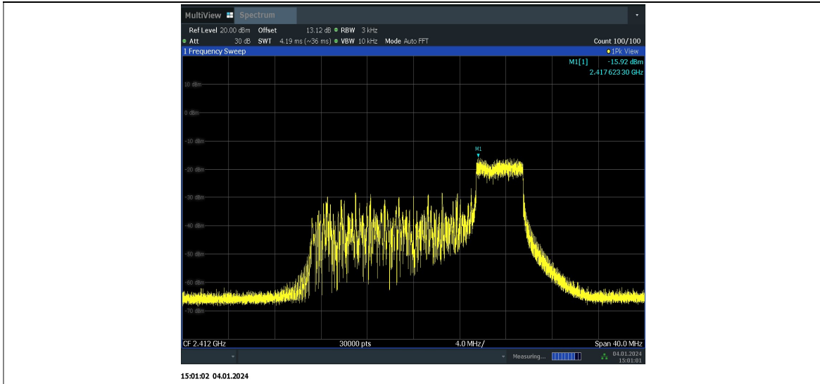
11AX20MIMO_Ant10_2412_106Tone_RU53
