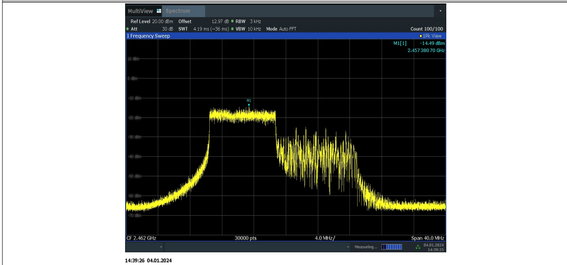
11AX20SISO_Ant10_2462_106Tone_RU54
