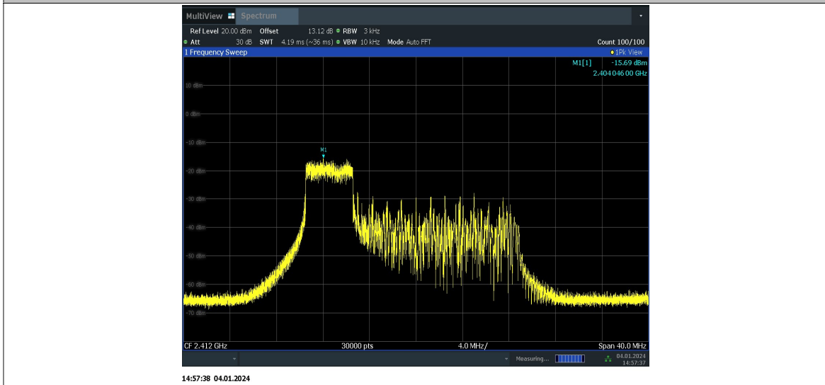
11AX20MIMO_Ant10_2412_52Tone_RU40
