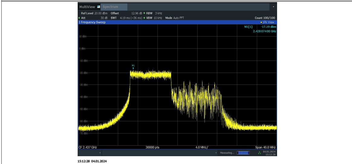
11AX20MIMO_Ant6_2437_106Tone_RU54
