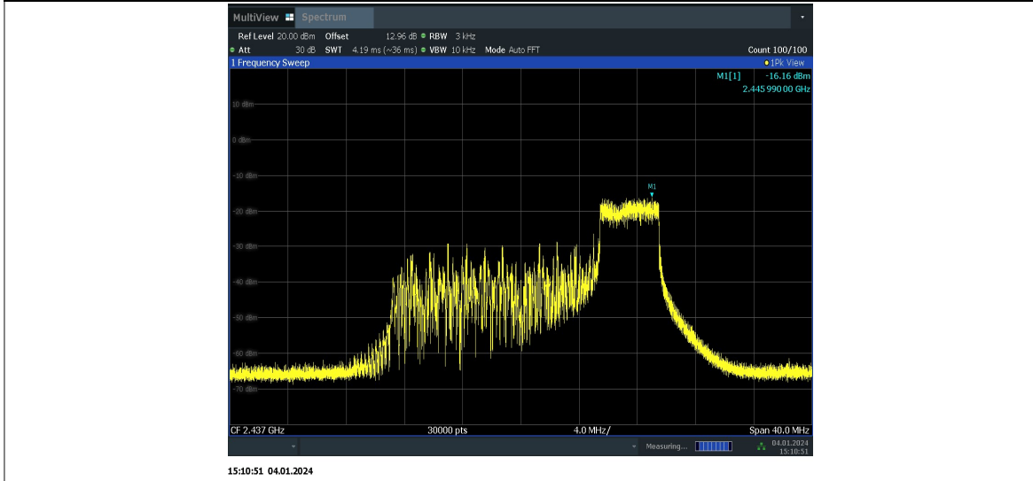
11AX20MIMO_Ant6_2437_106Tone_RU53
