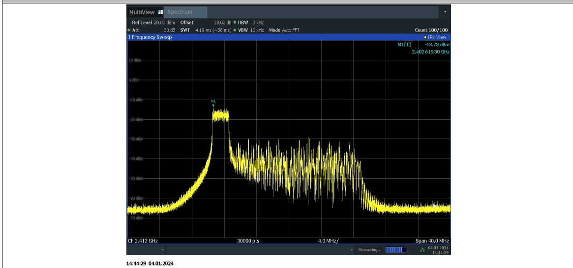
11AX20MIMO_Ant6_2412_26Tone_RU8
