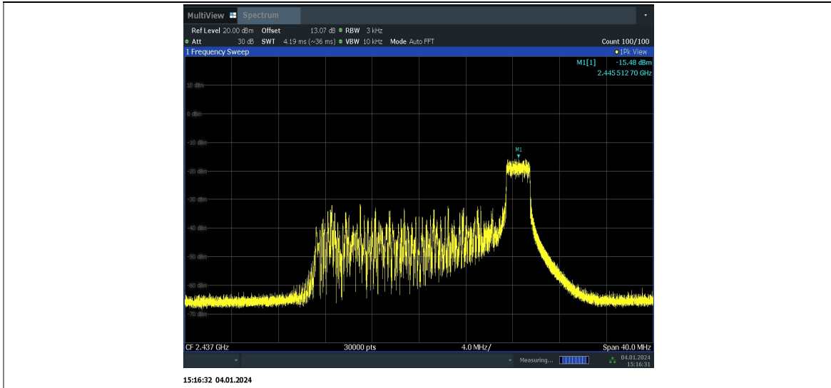
11AX20MIMO_Ant10_2437_52Tone_RU37
