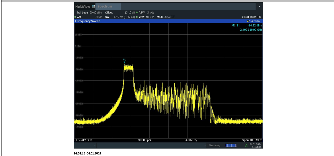
11AX20MIMO_Ant10_2412_26Tone_RU8
