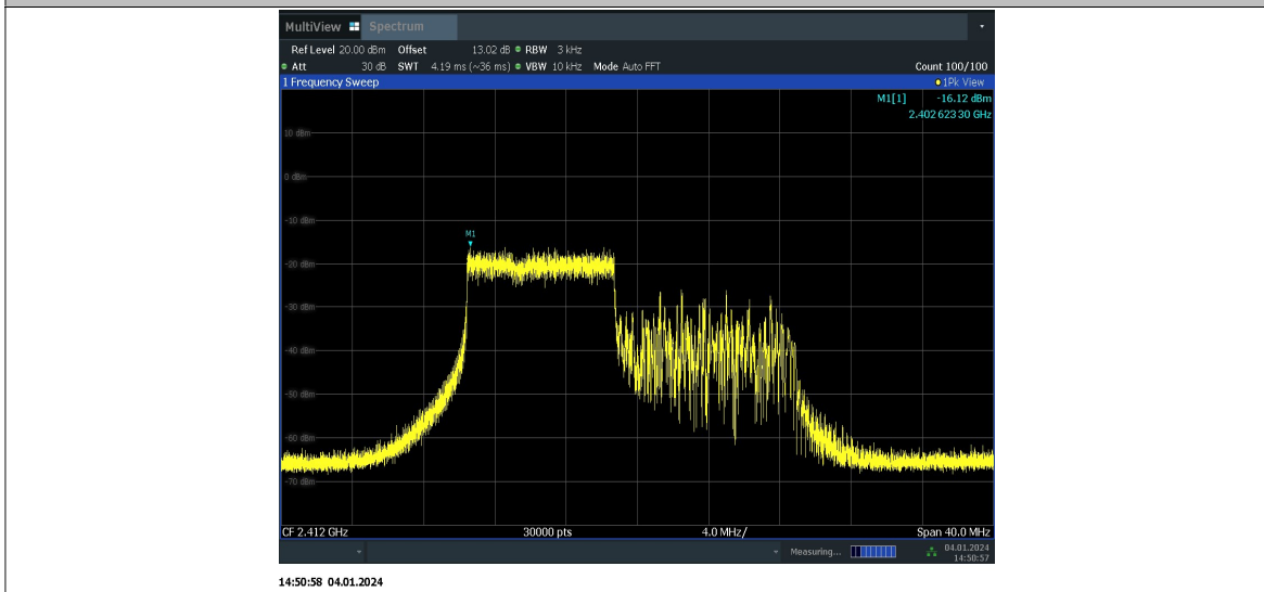
11AX20MIMO_Ant6_2412_106Tone_RU54
