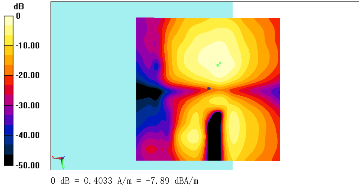
Fig B.13 T-Coil WCDMA 1900 -OTT
