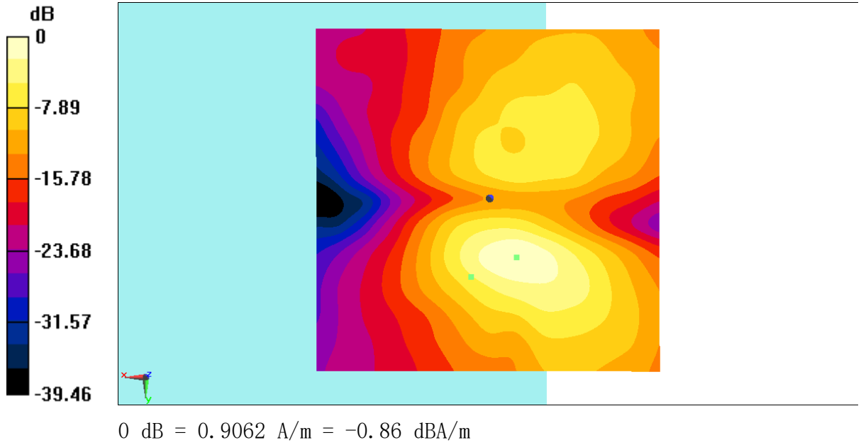
Fig B.13 T-Coil WCDMA 850
