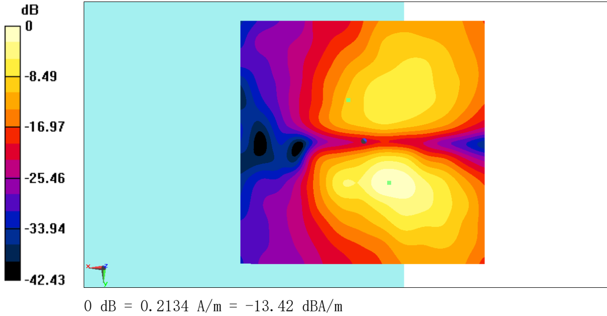
Fig B.9 T-Coil WiFi-2. 4G
