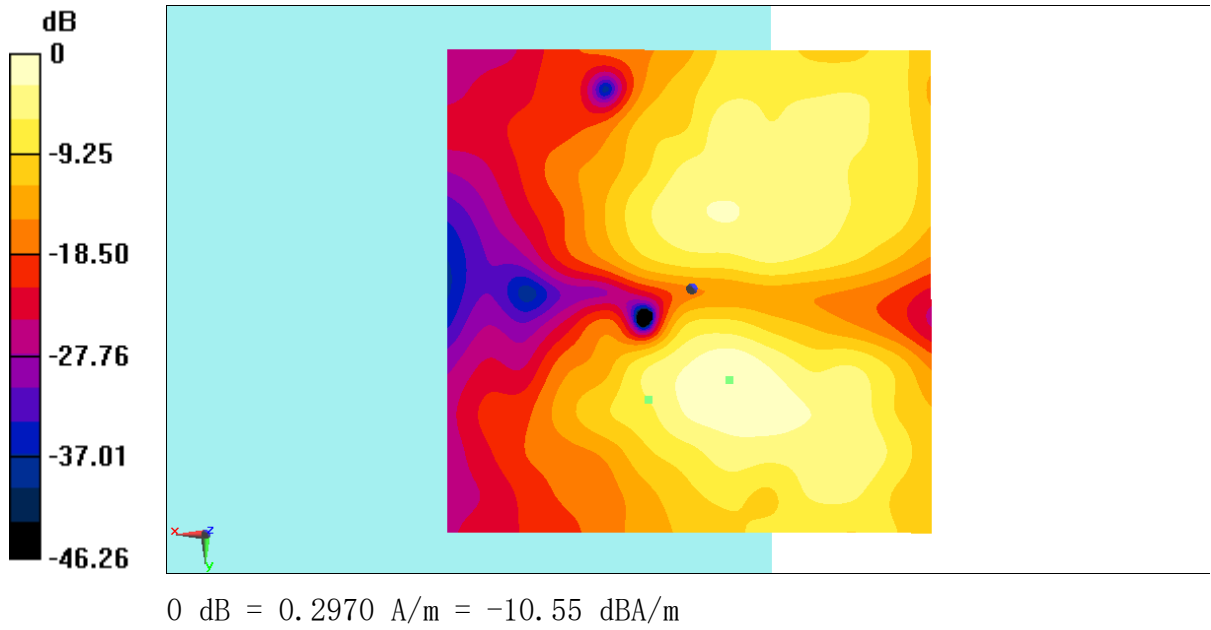
Fig B.19 T-Coil WiFi-2. 4G
