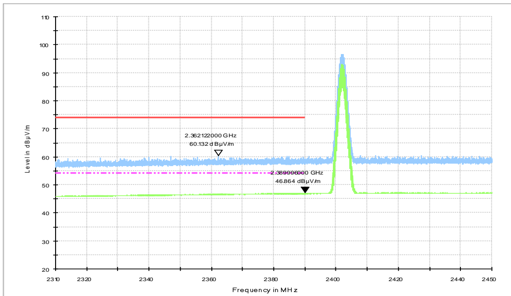
RE - Power-2.31GHz z 2.45GHz
