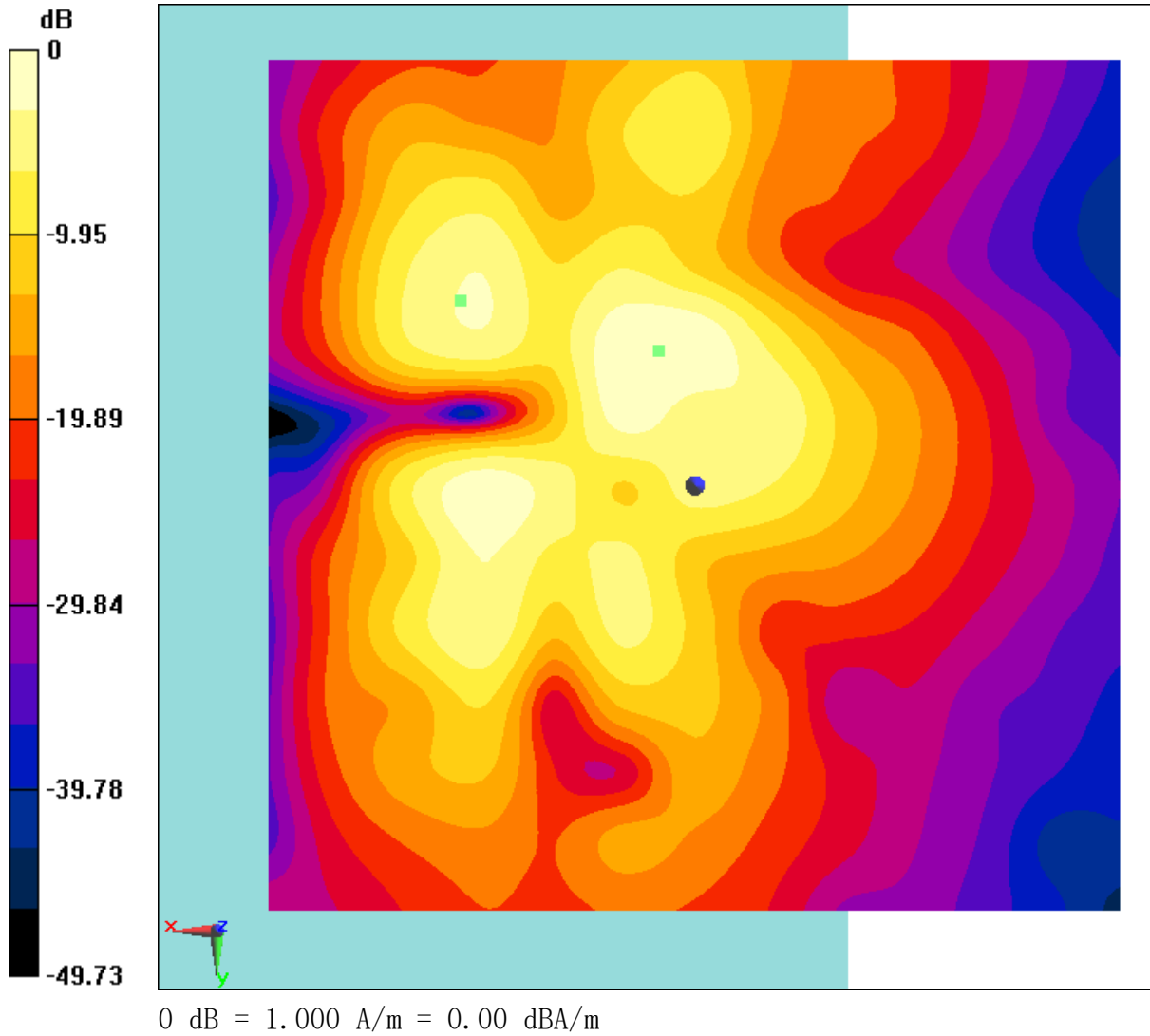
Fig B.23 T-Coil WiFi-2. 4G
