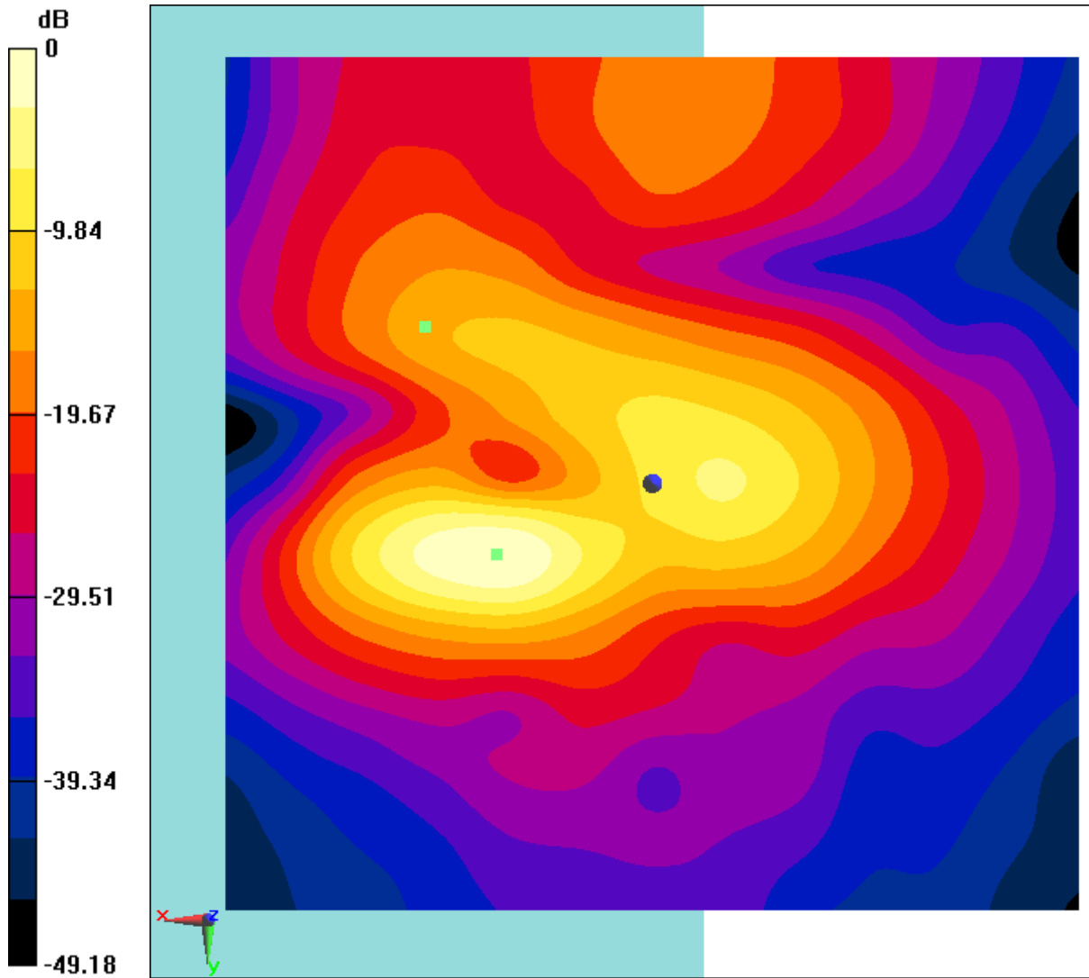
Fig B.7 T-Coil WCDMA 1900
