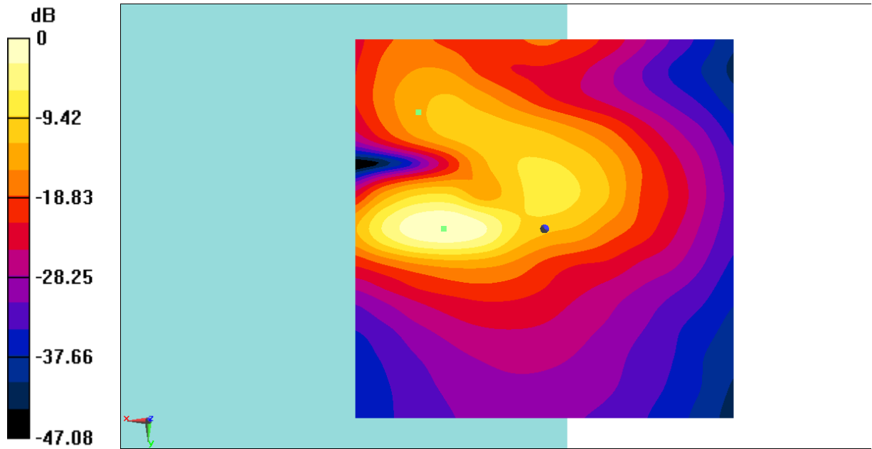
Fig B.7 T-Coil WCDMA 1900
