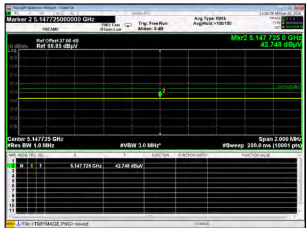
U-NII-1 11ax160 CH50 AV
