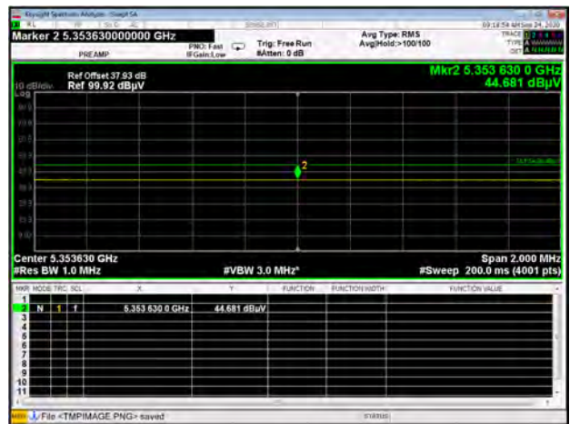
U-NII-2A 11ax20 CH64 AV
