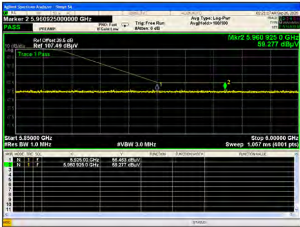
U-NII-3 11n40 CH142 Peak
