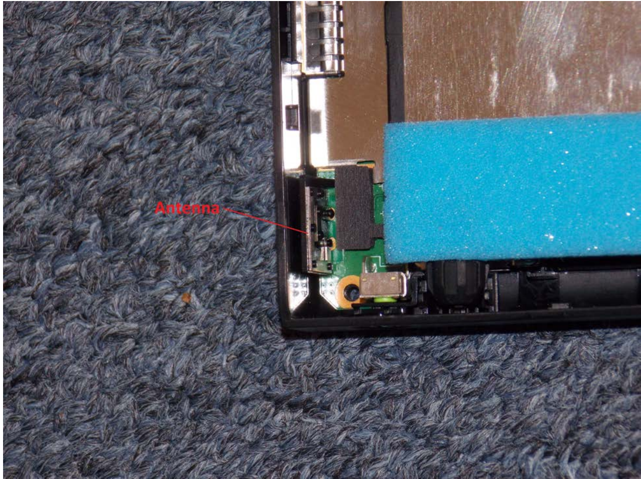
Antenna
