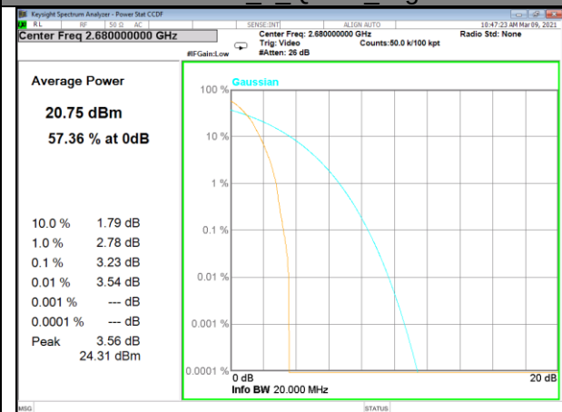
Band 41_1_Q16_High
