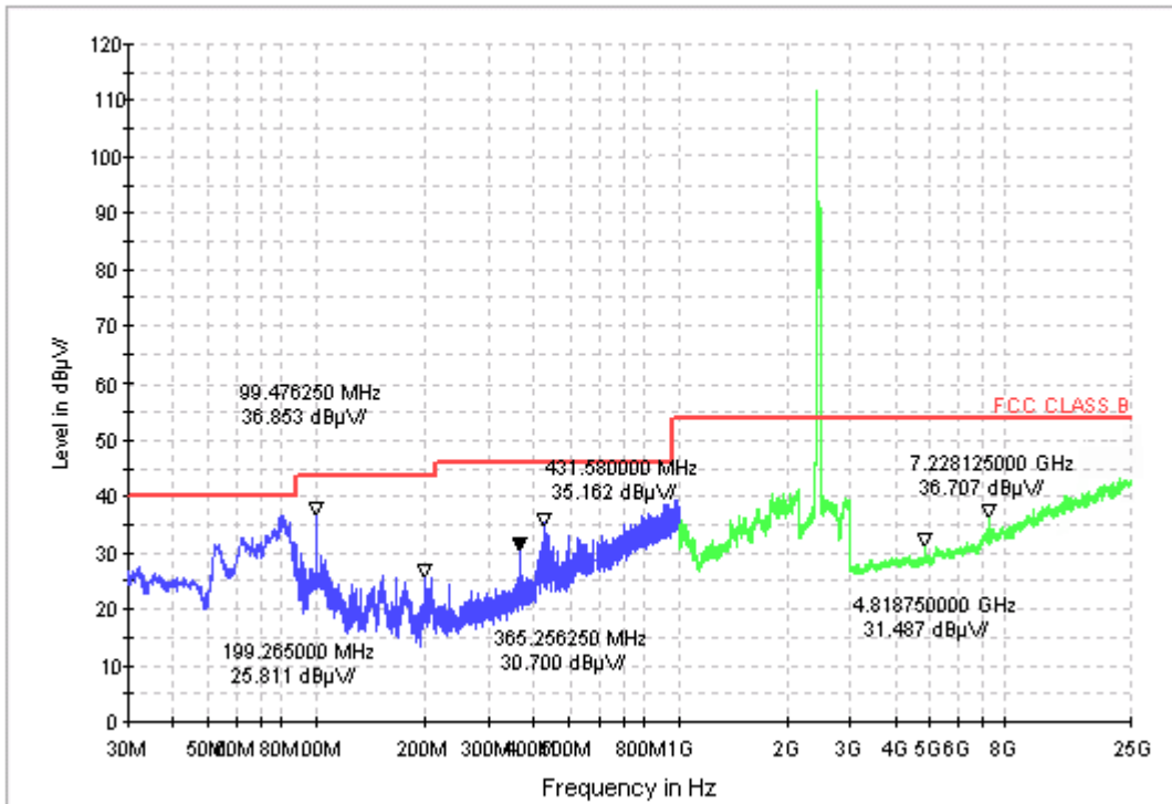
(Plot A.1: Antenna Horizontal)
