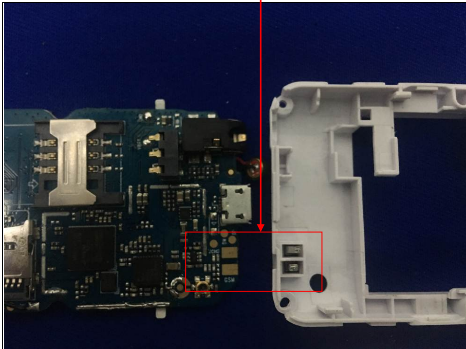
GSM Antenna
