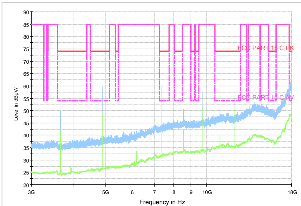
GFSK DH5 Channel 39 3-18GHz
