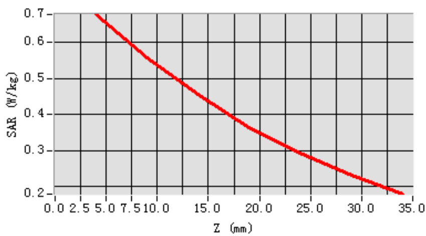
SAR, Z Axis Scan (X = -53, Y = -43)
