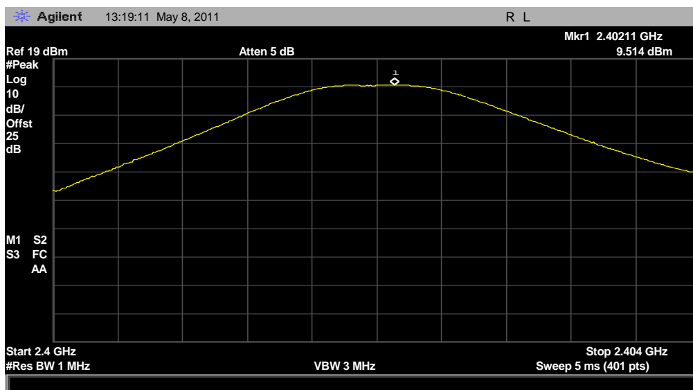
(Plot A: Channel = 2402)
