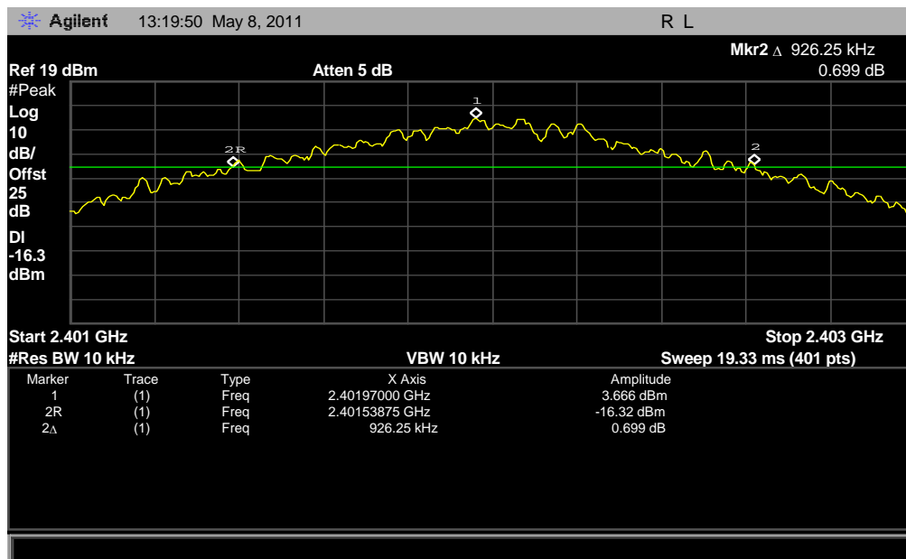
(Plot A: Channel = 2402)
