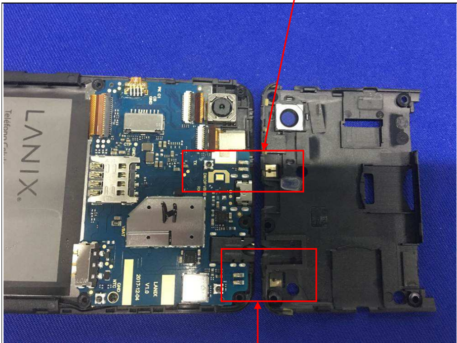
BT/WIFI Antenna
