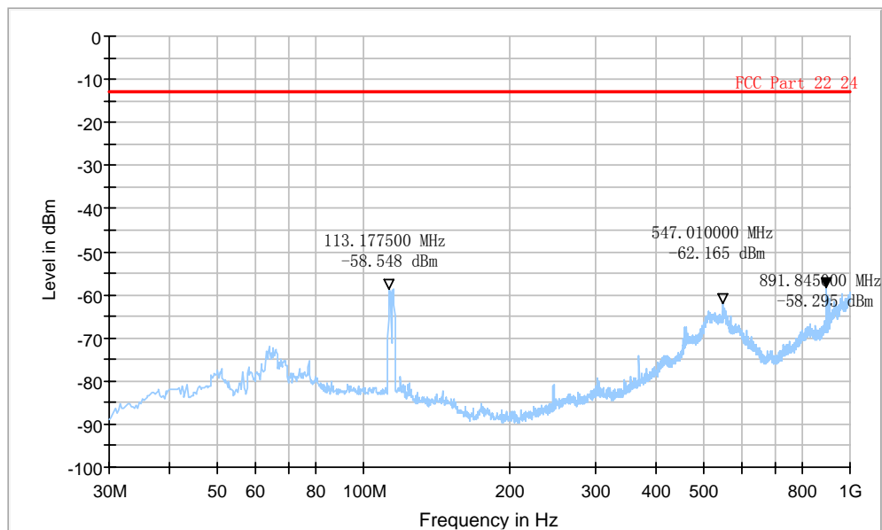
FCC 22H 24E 30M-1G
