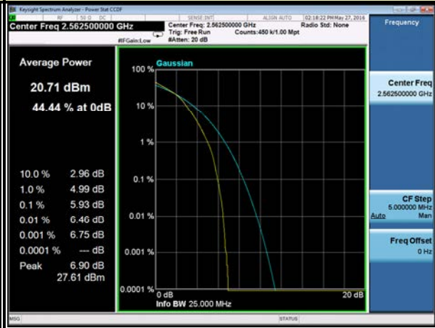
20MHz / 16QAM
