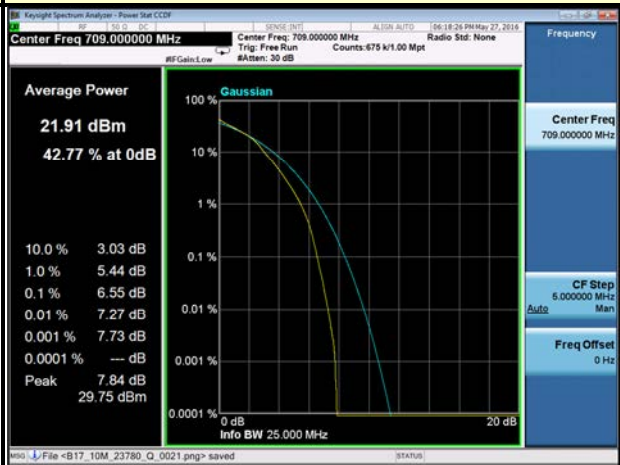
10MHz / 16QAM
