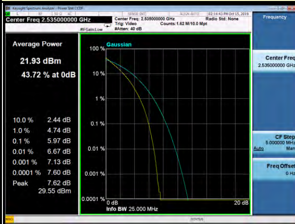
20MHz / QPSK
